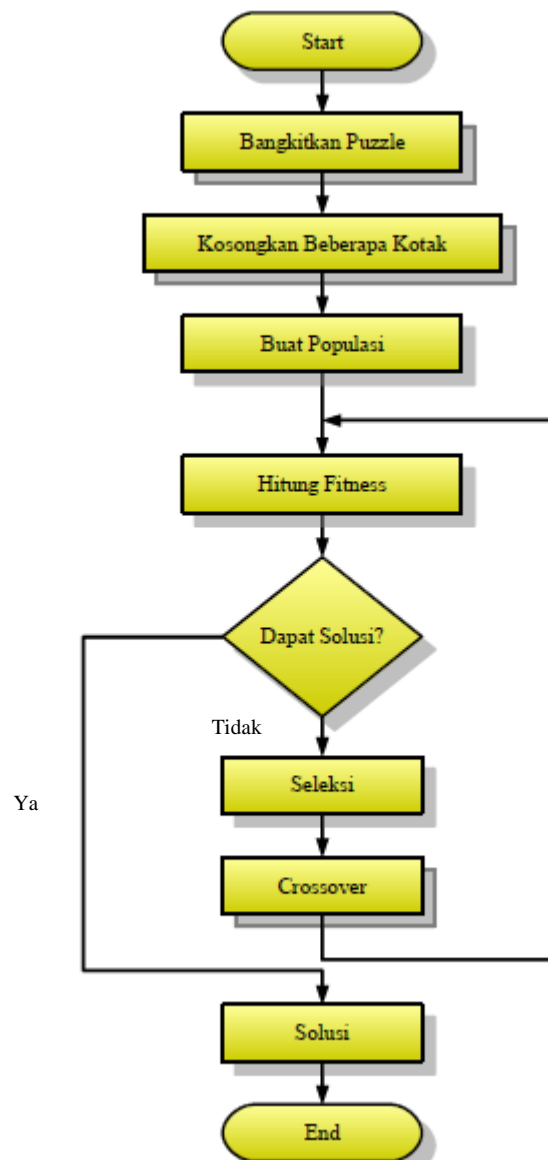
Gambar III.8. Flow Chart Algoritma Genetika pada Aplikasi Game Sudoku
