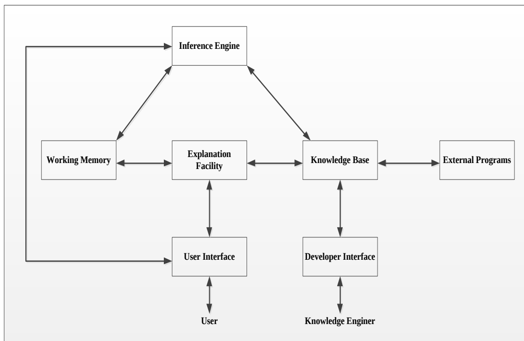
Gambar II.1.Arsitektur Sistem Pakar
