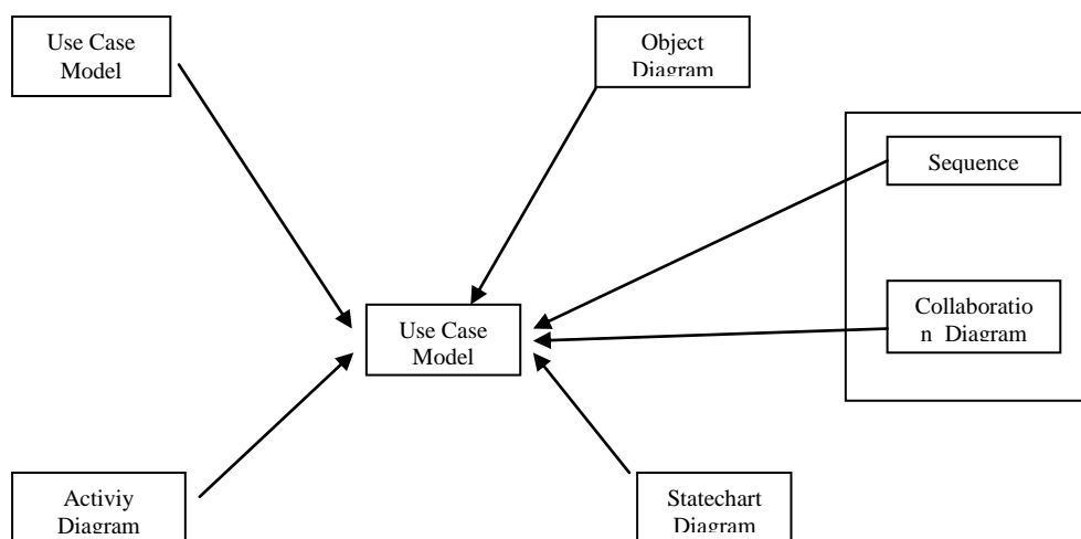
Gambar II.7. Hubungan Diagram Kelas Dengan Diagram UML lainnya
