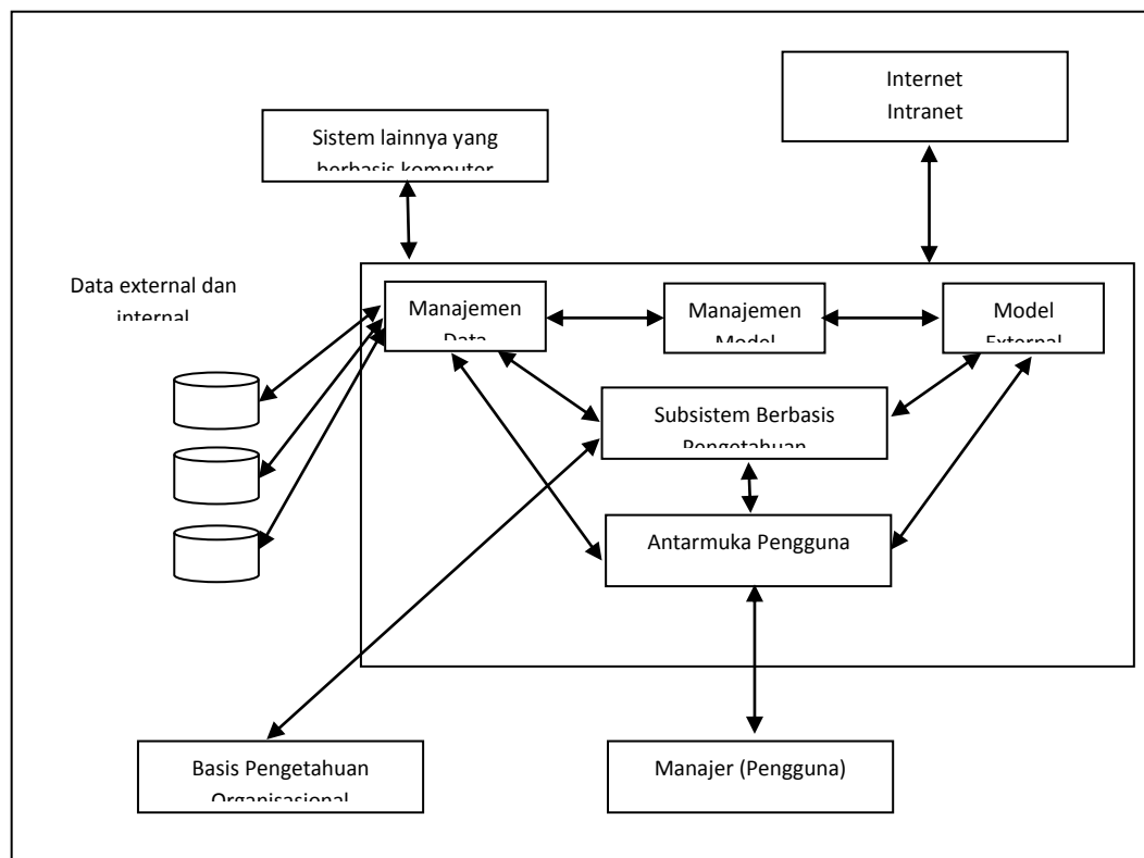
Gambar II.2. Arsitektur DSS (Sumber, Kusrini, M. Kom, 2007)
