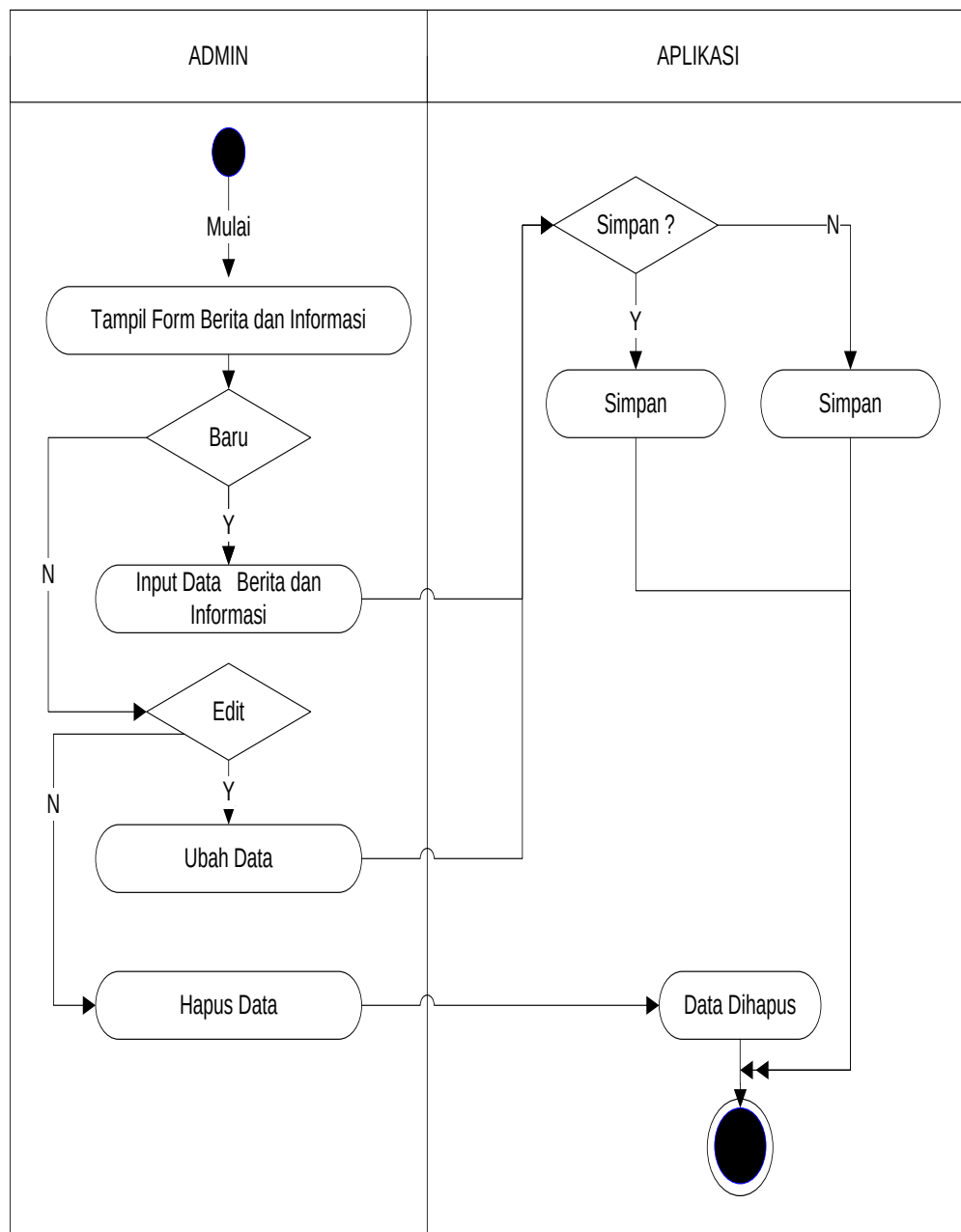
Gambar III.10. Diagram Activity Berita dan Informasi
