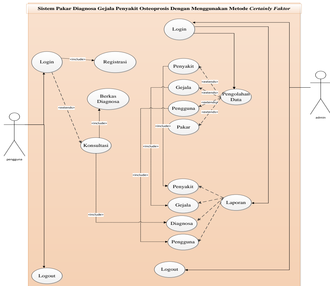
Gambar III.3. Use Case Diagram Sistem pakar mendiagnosa penyakit Osteoporosis Dengan Metode Certainty Factor
