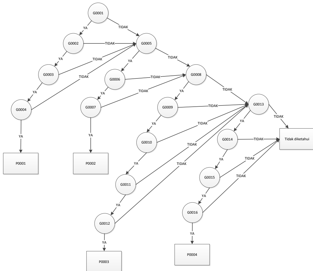
Gambar III.2. Pohon Aturan Sistem Pakar Diagnosa Gejala Penyakit Osteoporosis Dengan Menggunakan Metode Certainty Factor
