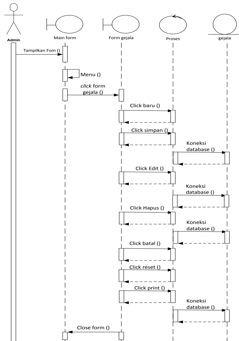
Gambar III.19. Sequence Diagram Data Daftar Pengguna
