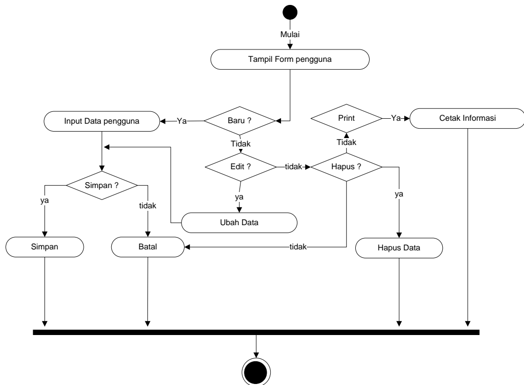
Gambar III.9. Activity Diagram Data Daftar Pengguna
