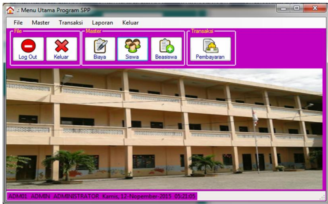
Gambar IV.2 Menu Utama
