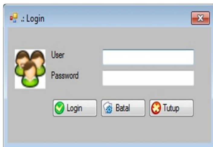
Gambar IV.1 Menu Login
