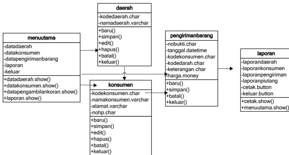
Gambar III.8 Class Diagram Laporan pada PT. Ekspedisi Muatan Kapal Laut
