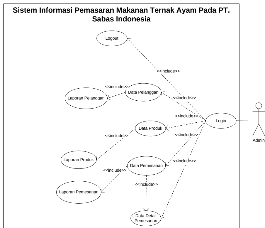
Gambar III.4 Use Case Sistem Informasi Pengolahan Makanan Ternak Ayam Pada PT. Sabas Indonesia
