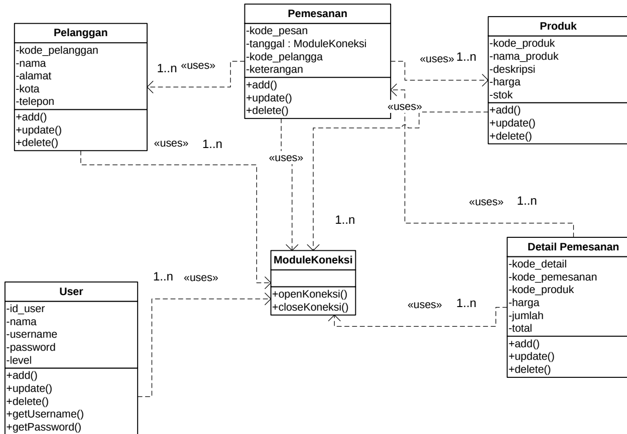
Gambar III.5 Class Diagram Sistem Informasi Pengolahan Makanan Ternak Ayam Pada PT. Sabas Indonesia Medan
