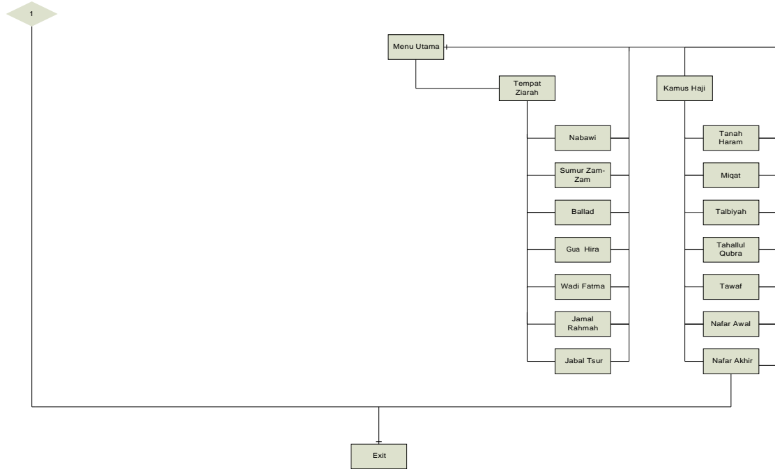
Gambar 2 Blok Diagram Aplikasi Tuntunan Haji ( Lanjutan )
