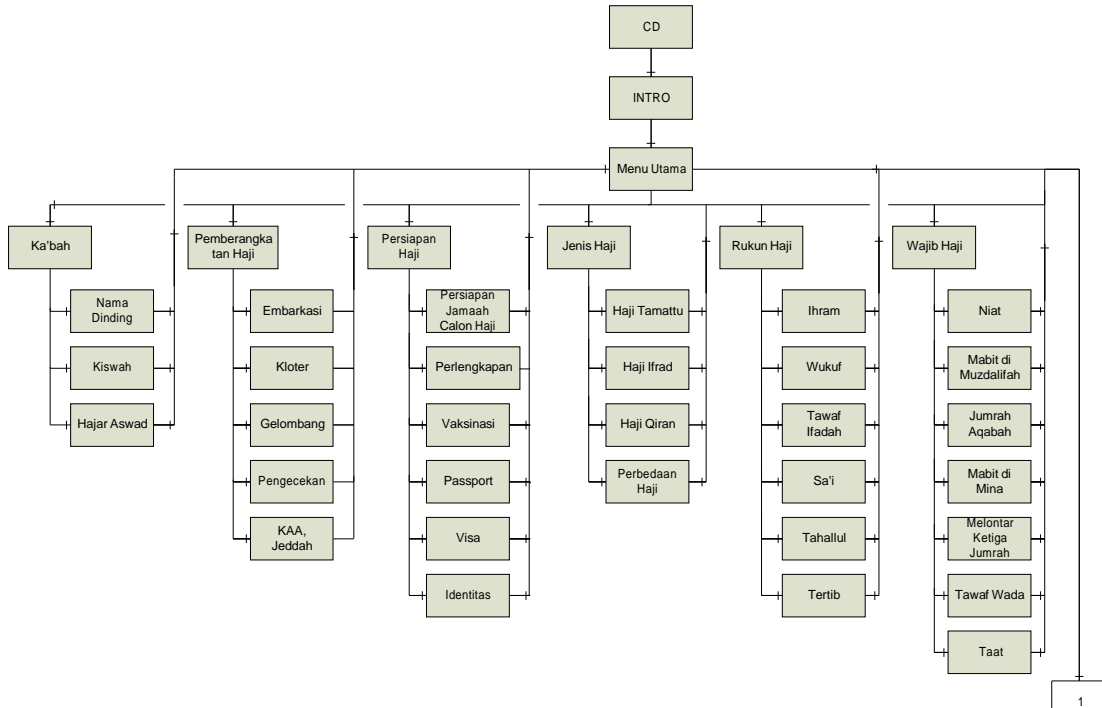
Gambar 1 Blok Diagram Aplikasi Tuntunan Haji
