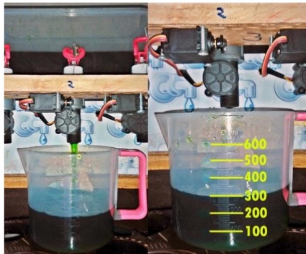
Gambar 8. Pengujian debit air Kran 2
