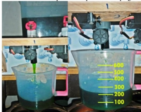
Gambar 7. Pengujian debit air Kran 1
