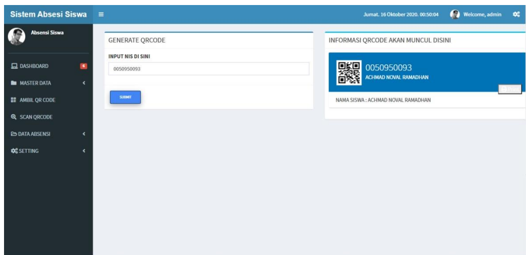
Gambar IV.8. Tampilan Ambil QR Code
