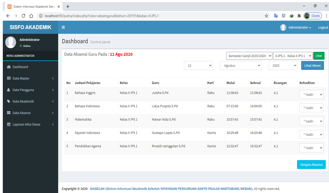
Gambar IV.20. Halaman Data Absensi Guru
