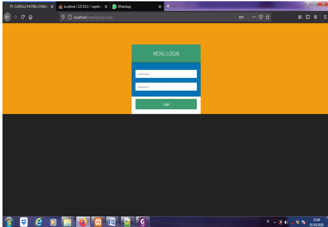
Gambar IV.1. Tampilan Login
