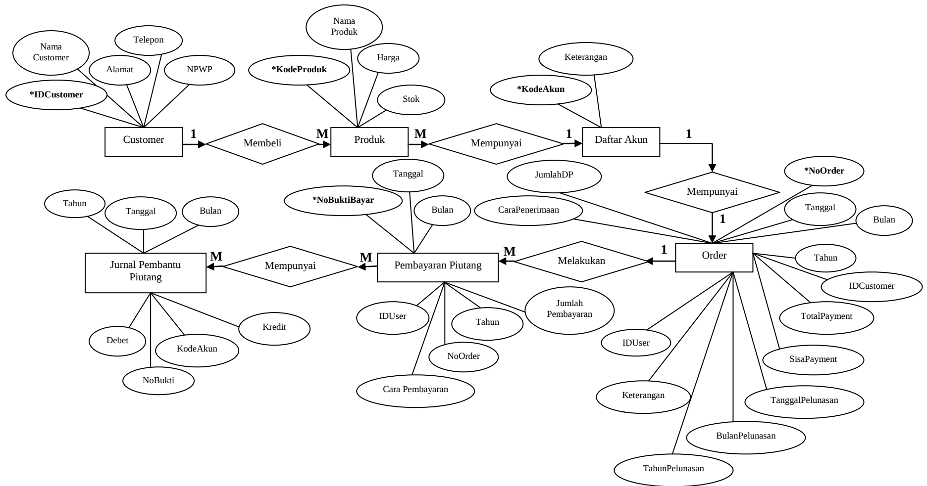
Gambar III.43. Entity Relationship Diagram (ERD) Perancangan Sistem Informasi Laporan Piutang Dagang Berbasis Client Server Pada PTPN III Medan Menggunakan VB. Net Dan MYSQL.
