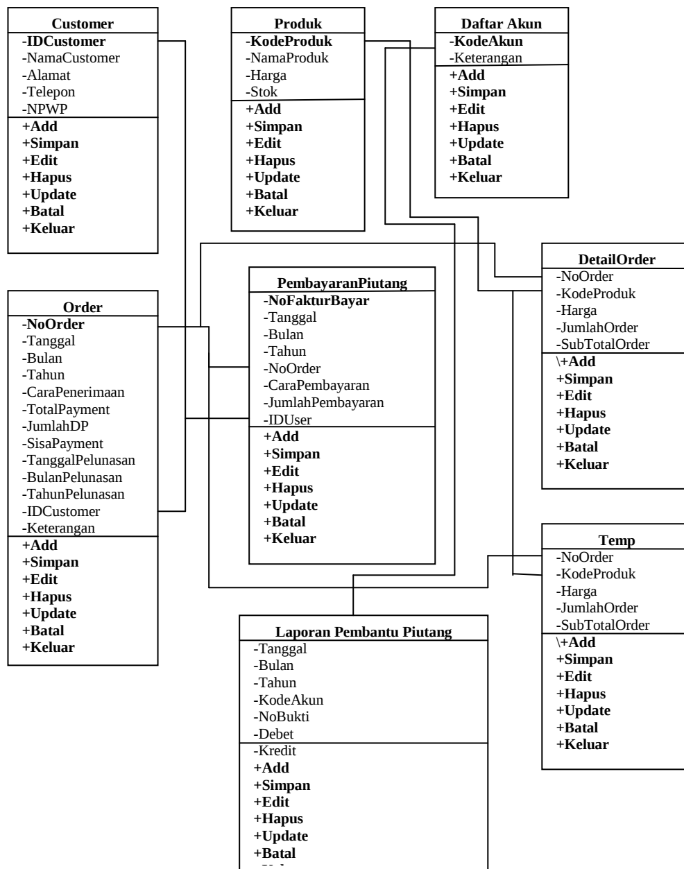
Gambar III.5. Class Diagram Perancangan Sistem Informasi Laporan Piutang Dagang Berbasis Client Server Pada PTPN III Medan Menggunakan VB. Net Dan MYSQL
