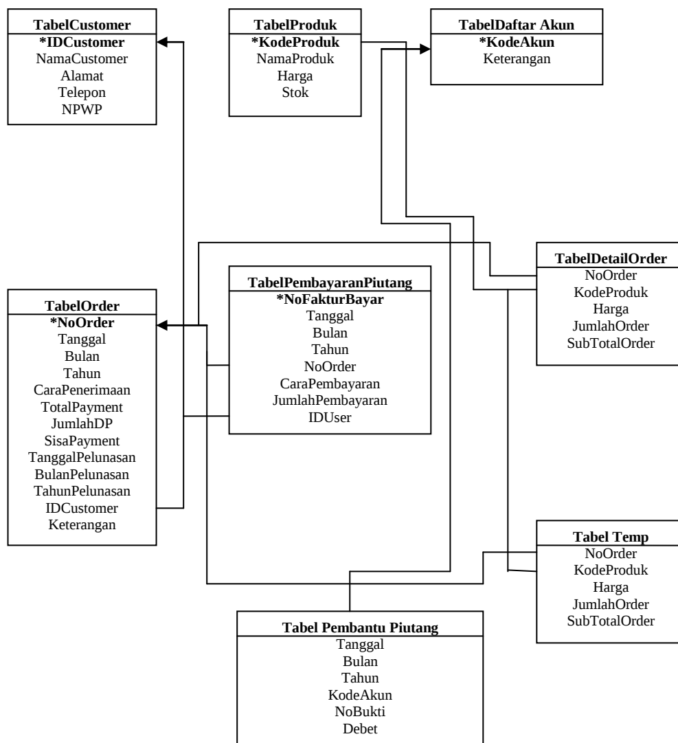
Gambar III.44. Relasi Antar Tabel Perancangan Sistem Informasi Laporan Piutang Dagang Berbasis Client Server Pada PTPN III Medan Menggunakan VB. Net Dan MYSQL.
