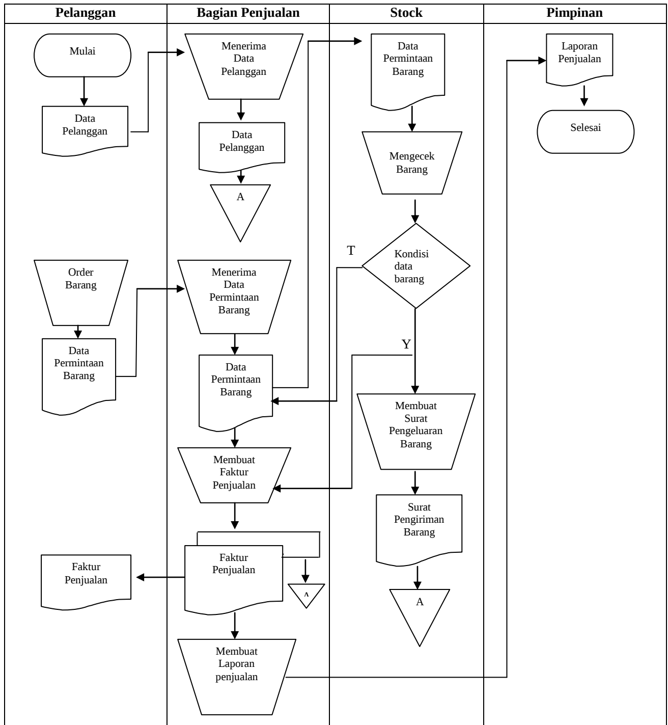
Gambar III.2. Flow Of Document Perancangan Sistem Informasi Laporan Piutang Dagang Berbasis Client Server Pada PTPN III Medan Menggunakan VB. Net Dan MYSQL Sumber : PTPN III Medan
