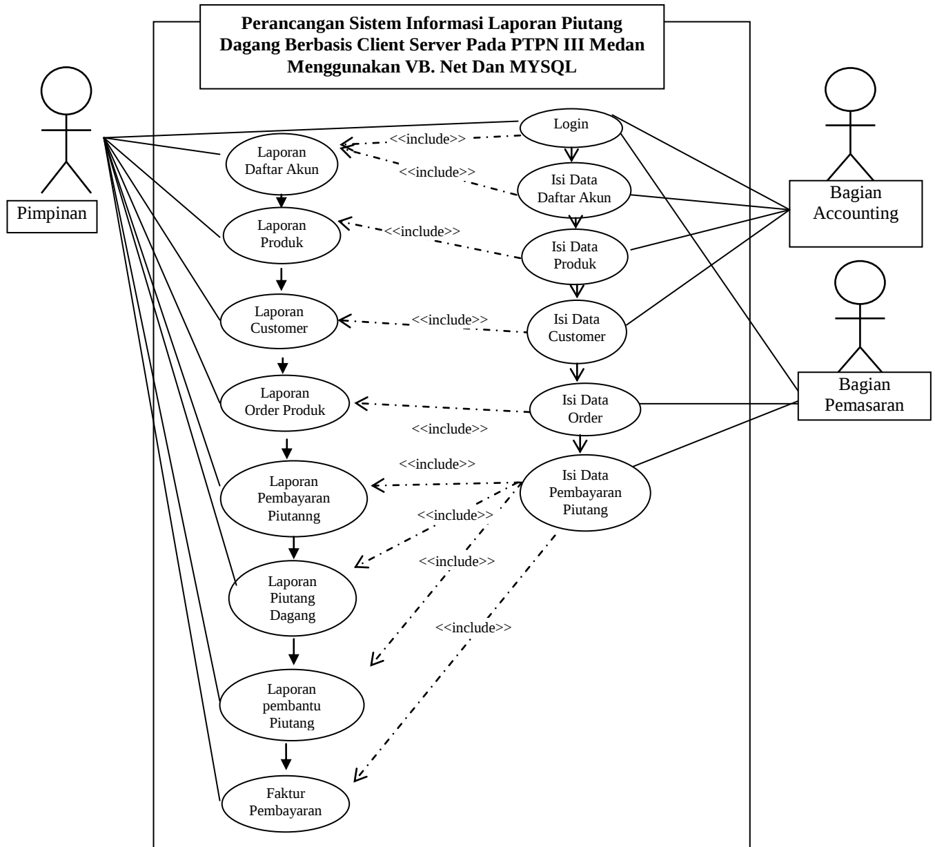
Gambar III.4. Use Case Perancangan Sistem Informasi Laporan Piutang Dagang Berbasis Client Server Pada PTPN III Medan Menggunakan VB. Net Dan MYSQL
