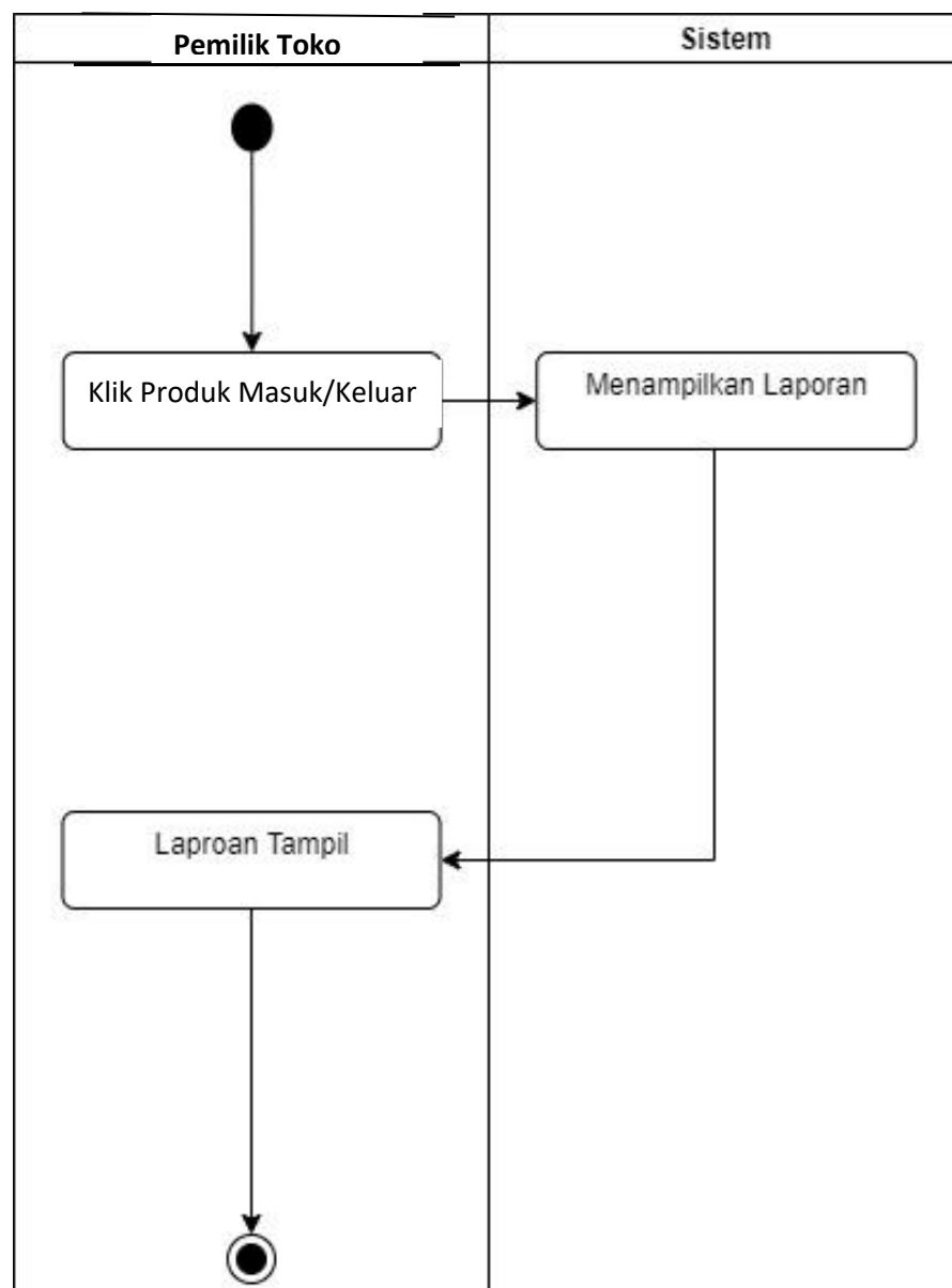
Gambar III.9. Activity Diagram Laporan Bagian Pemilik Toko
