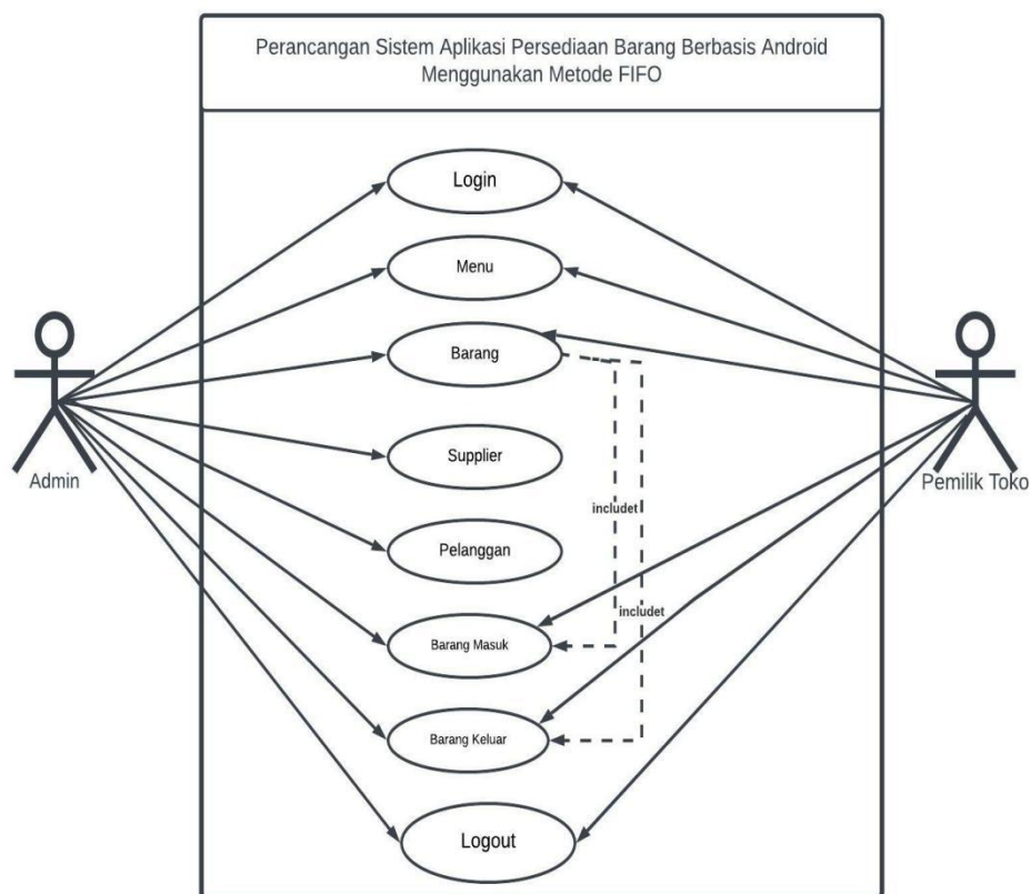
Gambar III.1. Use Case Perancangan Sistem Persediaan Barang
