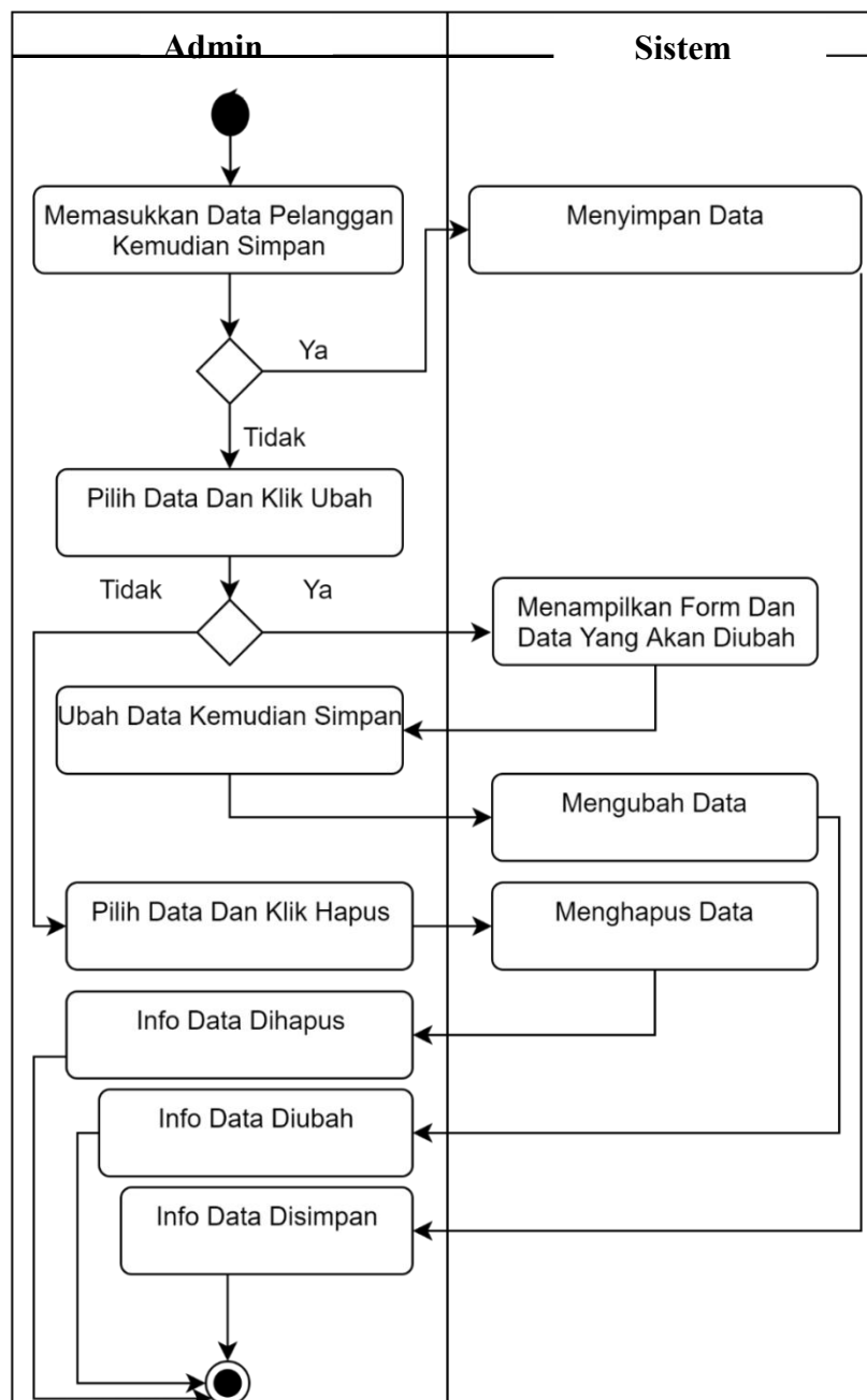
Gambar III.6. Activity Diagram Pelanggan Bagian Admin/Pemilik Toko
