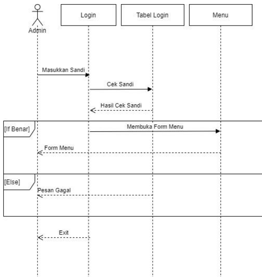
Gambar III.11. Sequence Diagram Login Bagian Admin/Pemilik Toko
