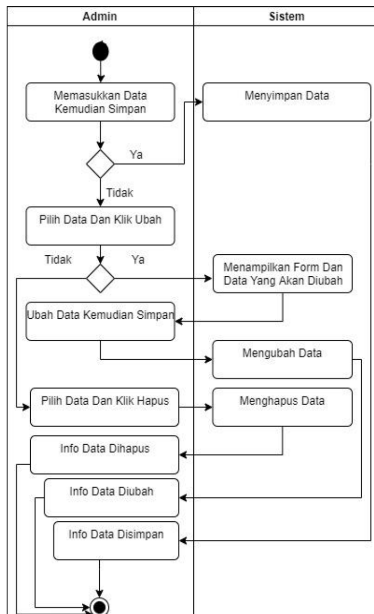
Gambar III.4. Activity Diagram Barang Bagian Admin/Pemilik Toko
