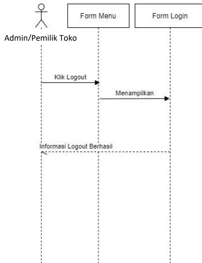
Gambar III.18. Sequence Diagram Logout Bagian Admin/Pemilik Toko
