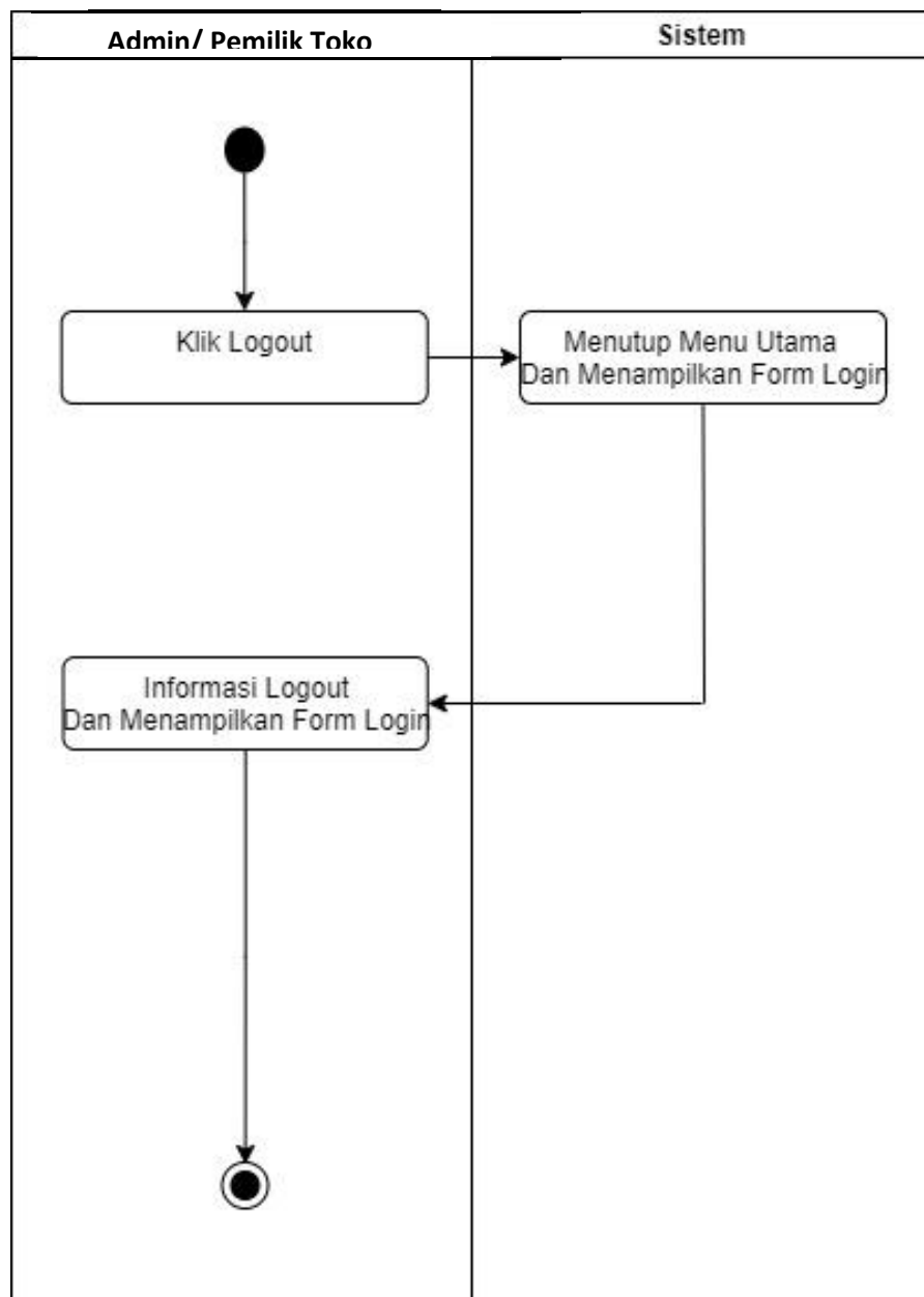
Gambar III.10. Activity Diagram Logout Bagian Admin/Pemilik Toko
