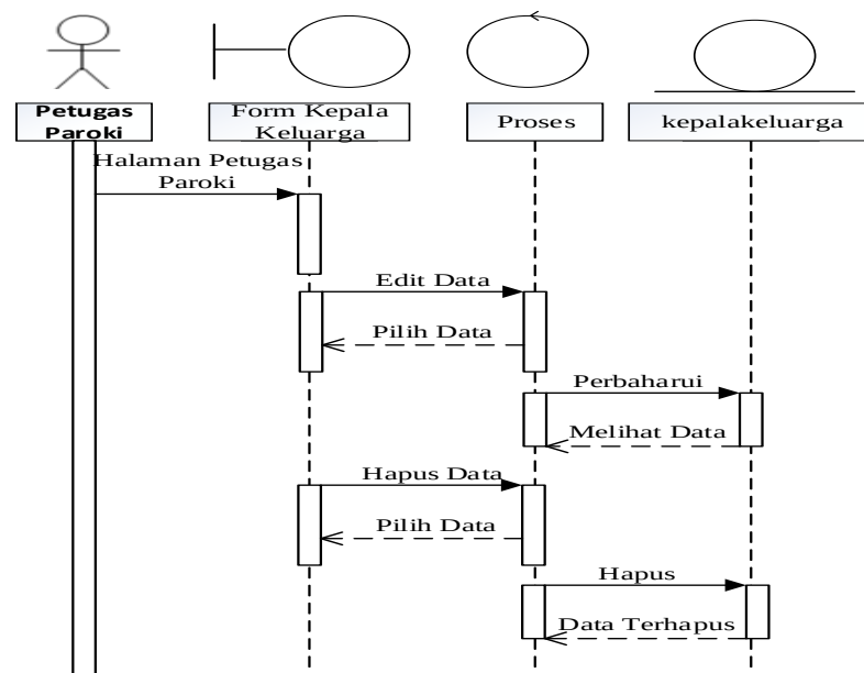
Gambar III.30. Sequence Diagram form Data Kepala Keluarga
