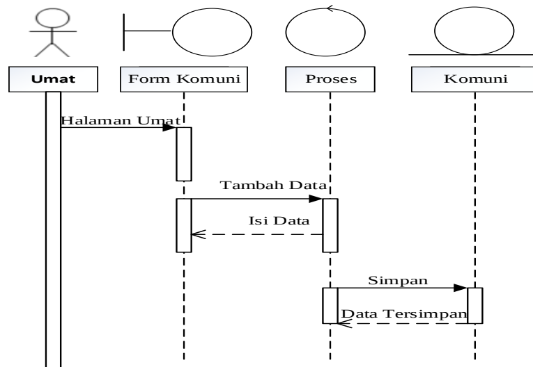
Gambar III.25. Sequence Diagram pada form Data Komuni
