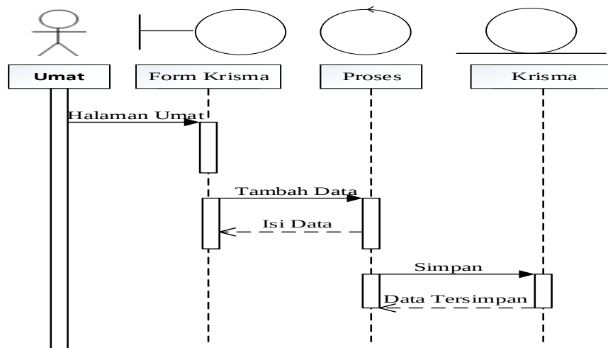
Gambar III.26. Sequence Diagram pada form Data Krisma
