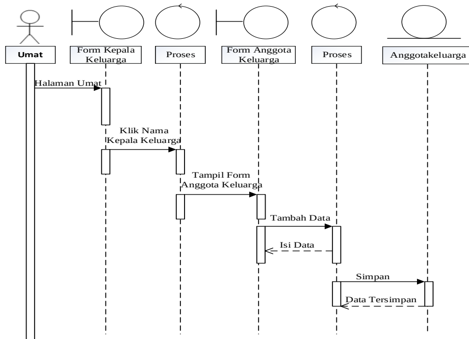
Gambar III.23. Sequence Diagram pada form Data Anggota Keluarga
