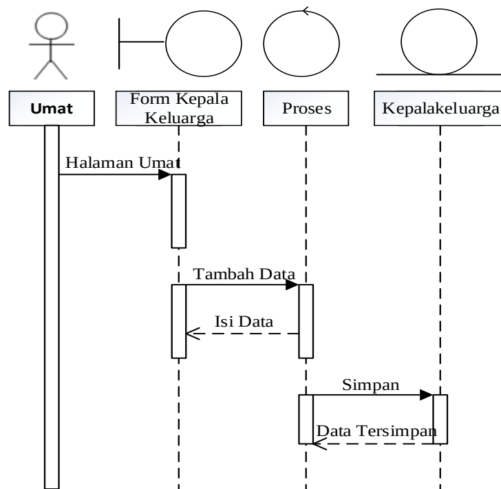
Gambar III.22. Sequence Diagram pada form Data Kepala Keluarga
