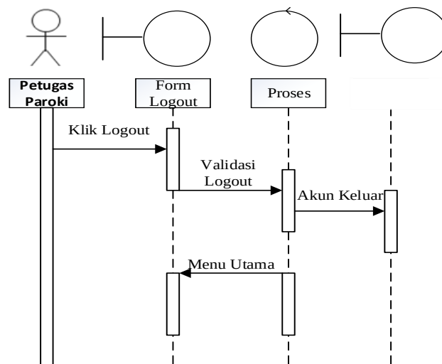
Gambar III.35. Sequence Diagram pada form logout petugas paroki
