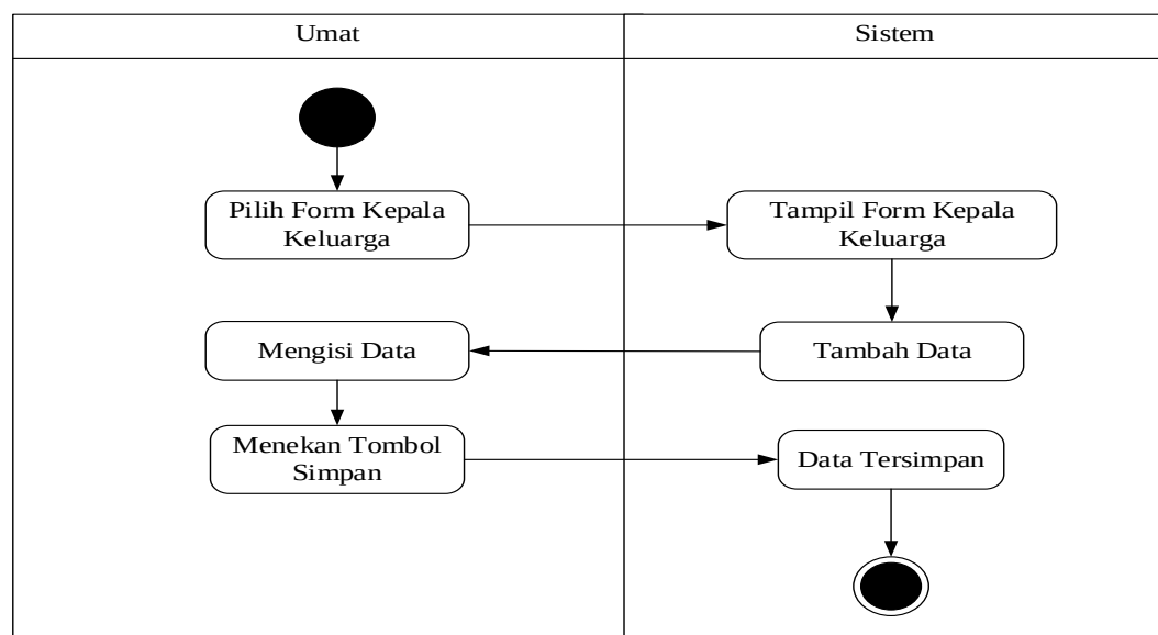
Gambar III.6. Activity Diagram Data Kepala Keluarga
