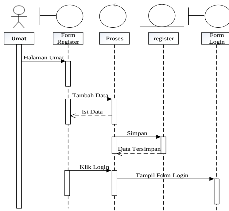
Gambar III.20. Sequence Diagram pada form registrasi
