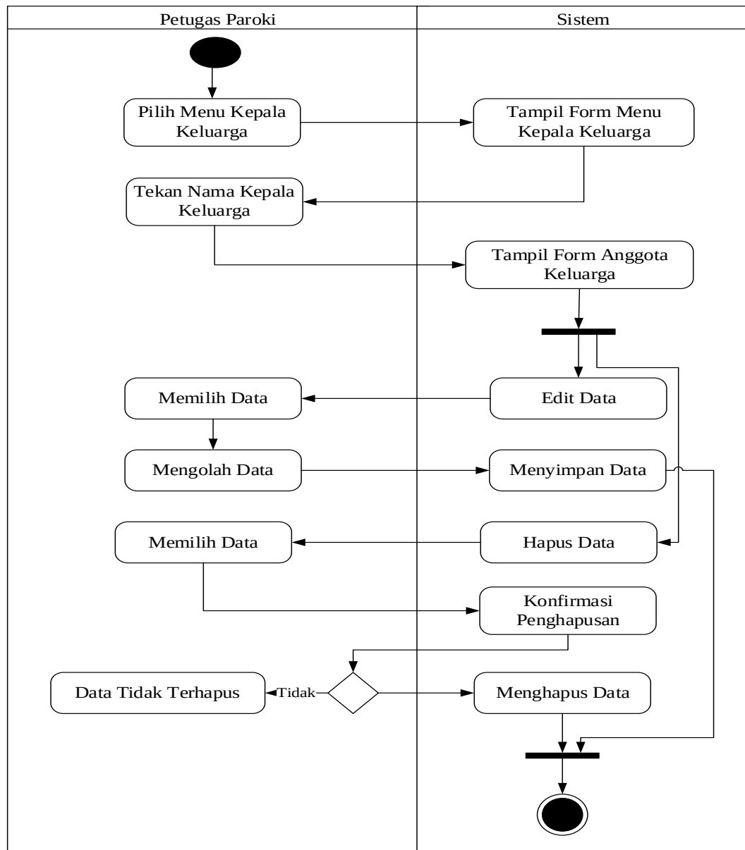
Gambar III.15. Activity Diagram Data Anggota Keluarga
