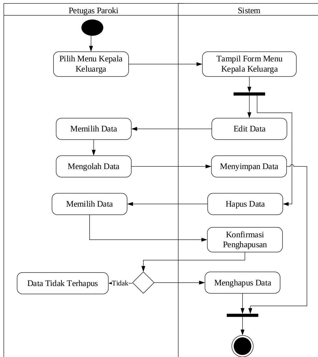
Gambar III.14. Activity Diagram Data Kepala Keluarga
