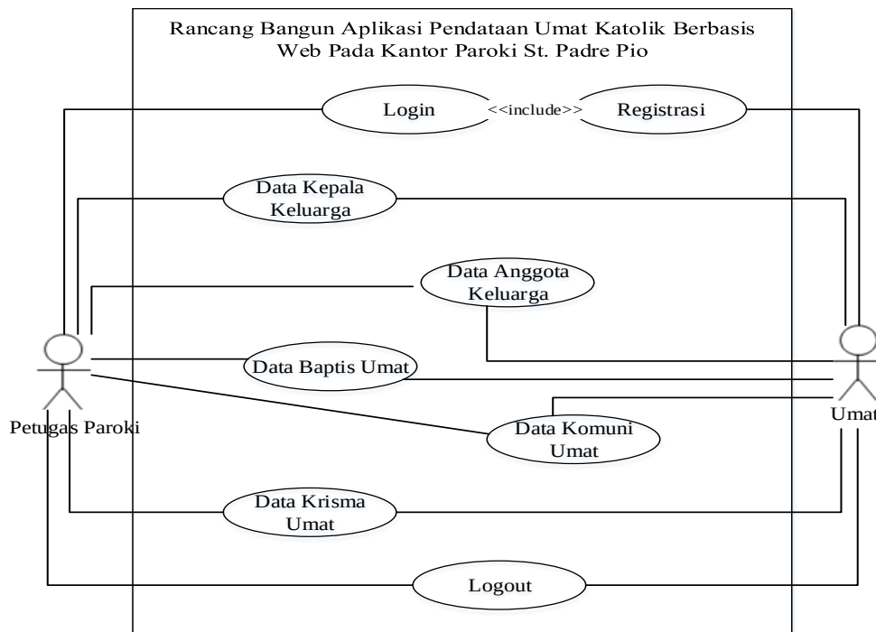
Gambar III.2. Use case Diagram Rancang Bangun Aplikasi Pendataan Umat Katolik Berbasis Web Pada Kantor Paroki St. Padre Pio
