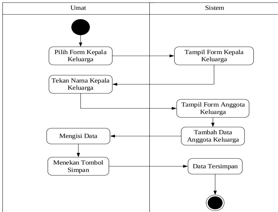
Gambar III.7. Activity Diagram Data Anggota Keluarga
