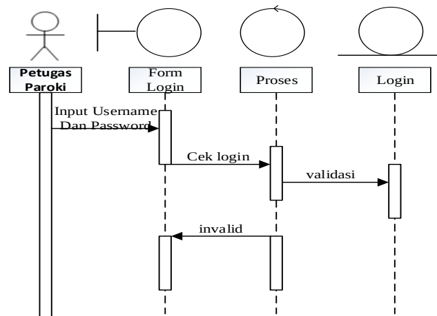
Gambar III.29. Sequence Diagram pada form login petugas paroki
