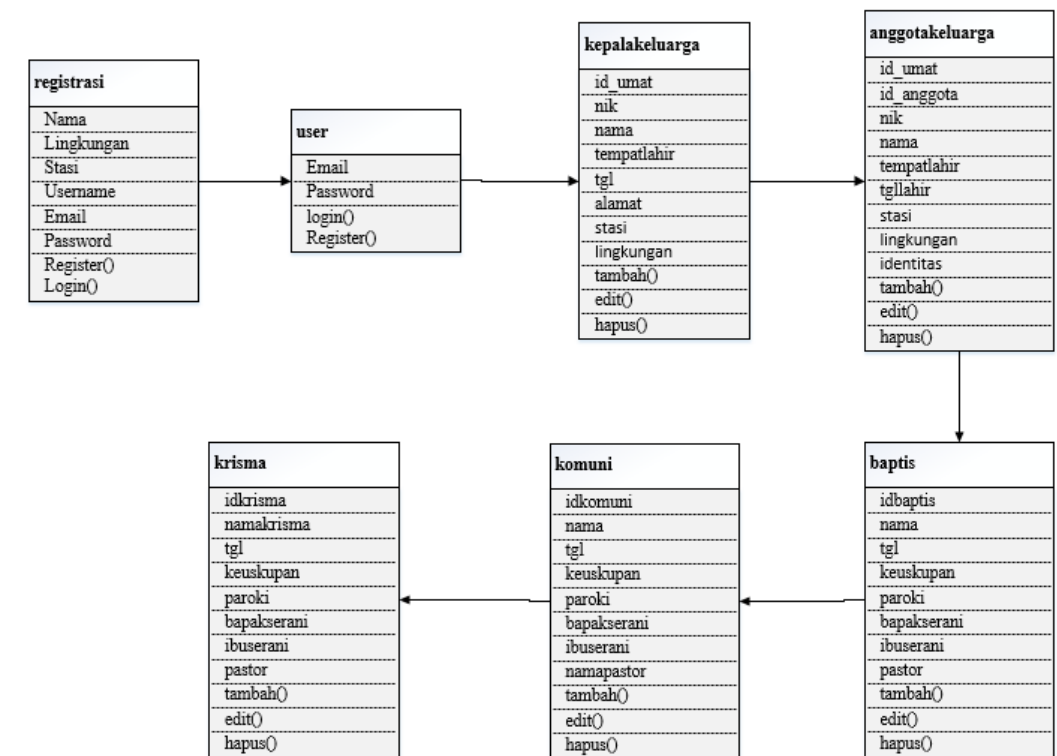
Gambar III.3. Class Diagram Rancang Bangun Aplikasi Pendataan Umat
