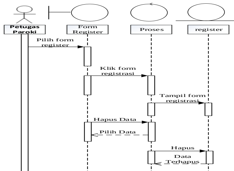
Gambar III.28. Sequence Diagram pada form data registrasi
