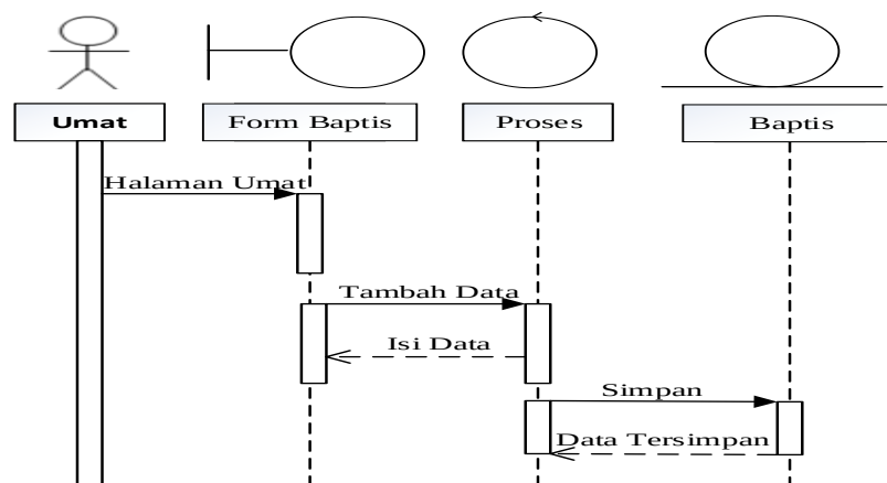
Gambar III.24. Sequence Diagram pada form Data Baptis
