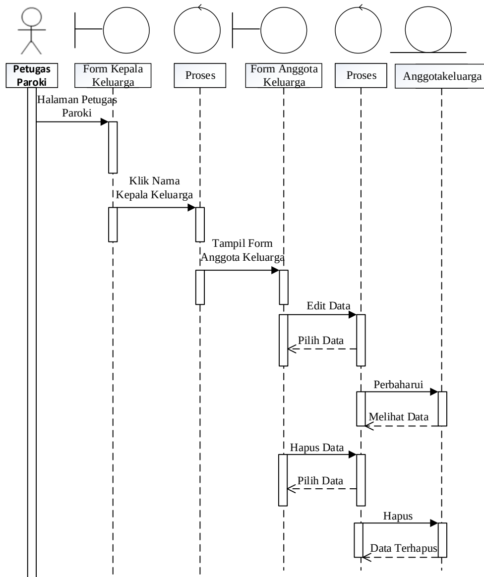
Gambar III.31. Sequence Diagram form Data Anggota Keluarga
