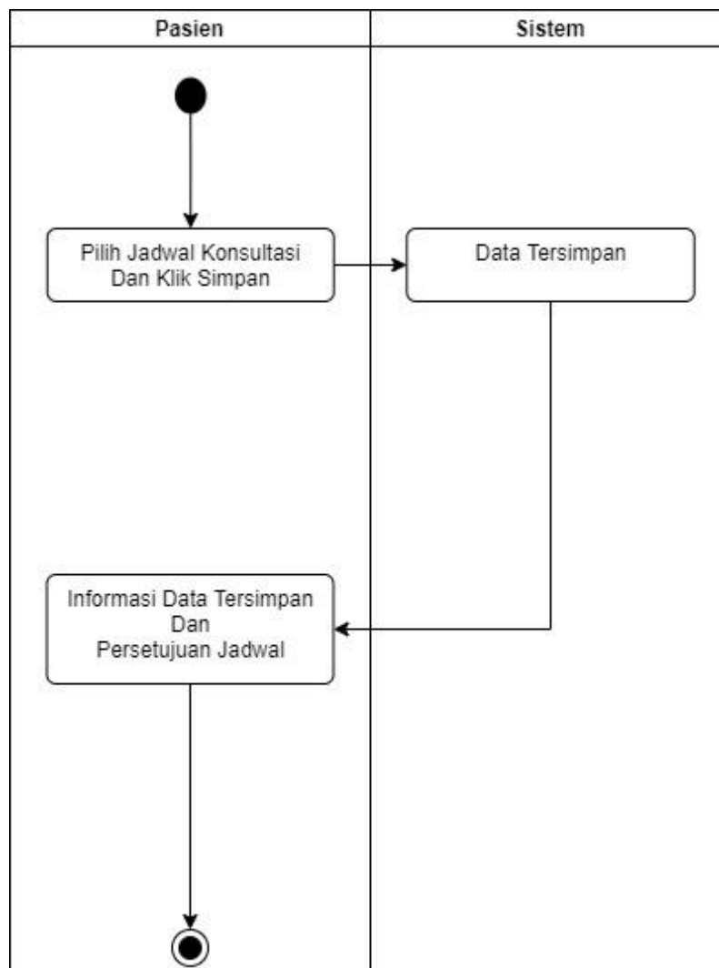
Gambar III.13. Activity Diagram Penjadwalan Konsultasi
