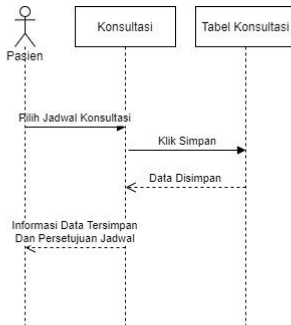
Gambar III.25. Sequence Diagram Penjadwalan Konsultasi
