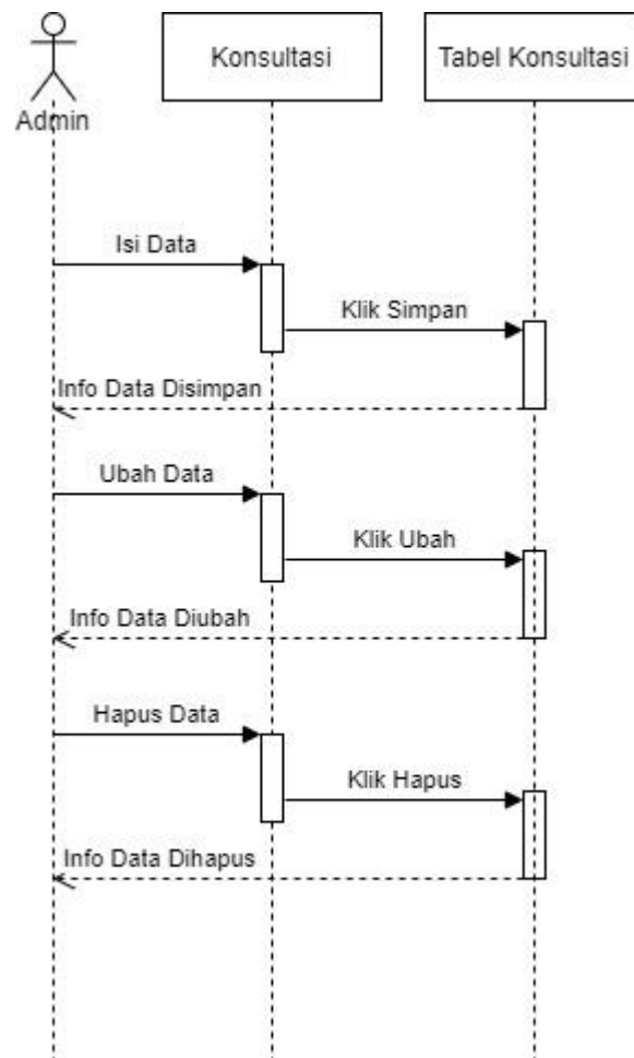
Gambar III.19. Sequence Diagram Penjadwalan Konsultasi
