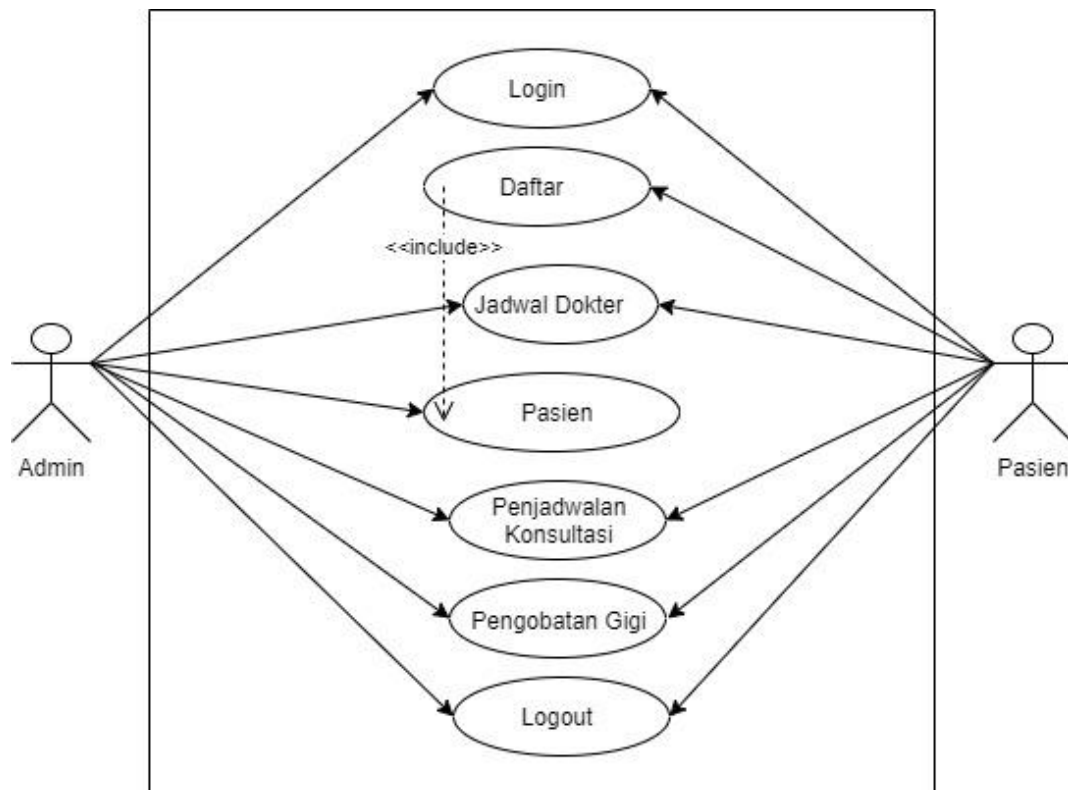
Gambar III.2. Use Case Perancangan Aplikasi Penjadwalan Konsultasi Dan Pengobatan Gigi Berbasis Web Dan Android Di Klinik Model Indah
