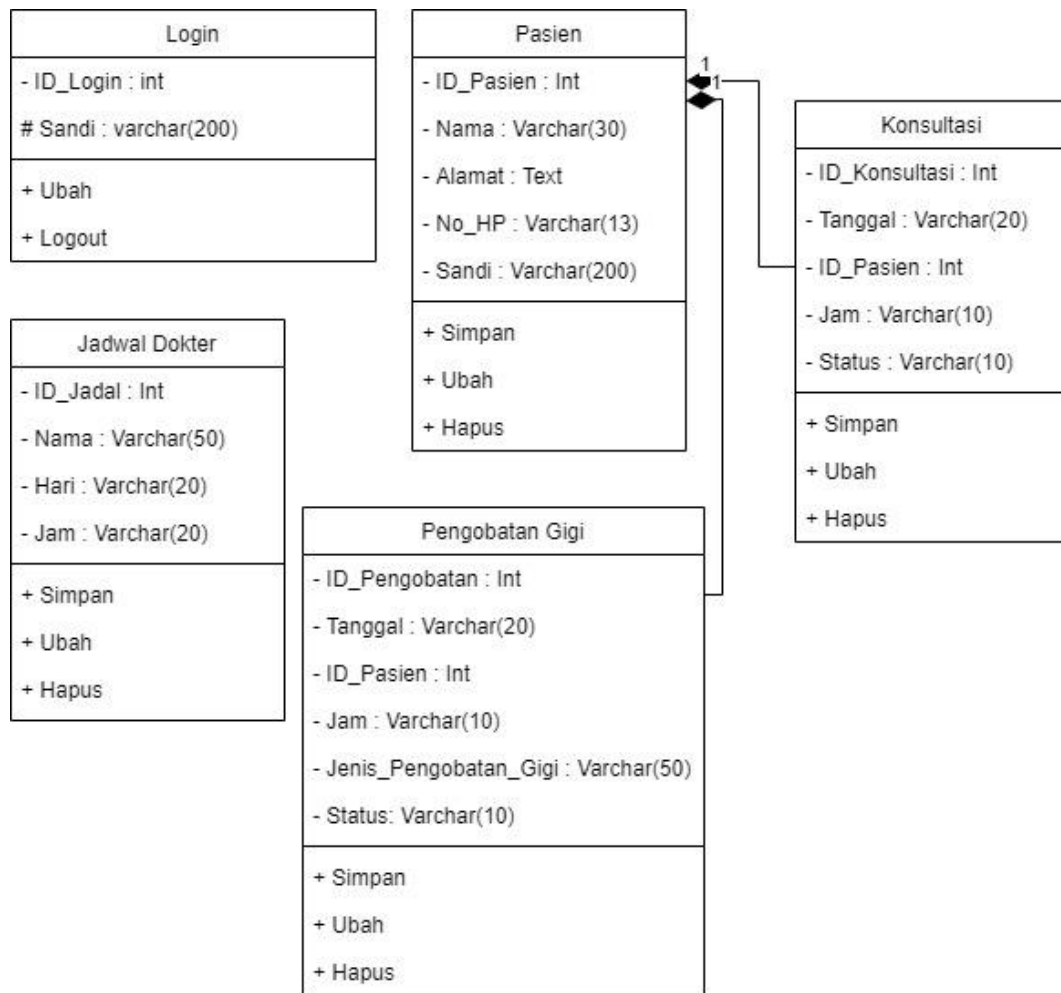
Gambar III.3. Class Diagram Perancangan Aplikasi Penjadwalan Konsultasi Dan Pengobatan Gigi Berbasis Web Dan Android Di Klinik Model Indah
