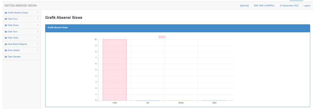
GambarIV.1.3.Tampilanformgrafik absensi
