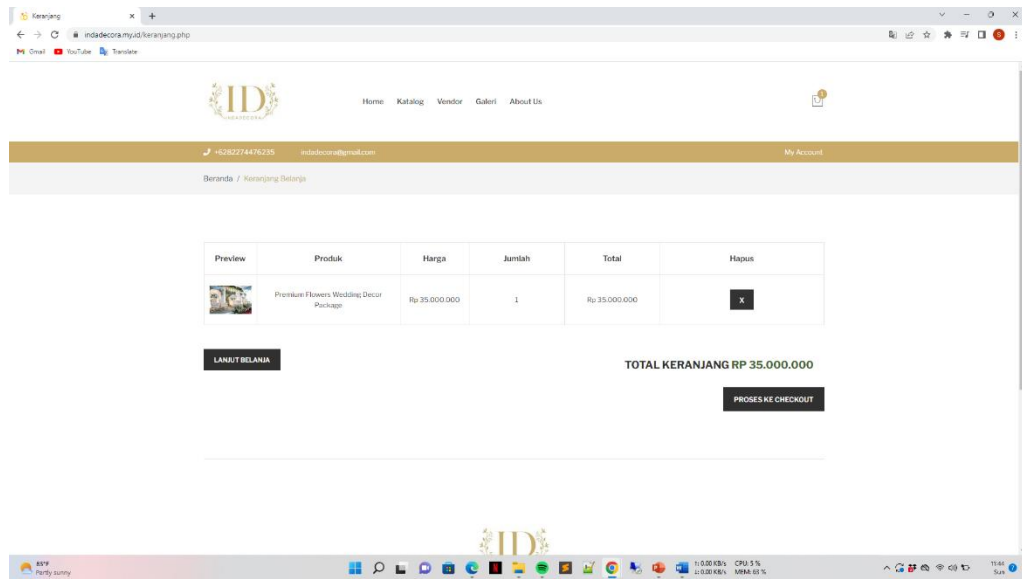
Gambar IV.9 Tampilan Pemesanan
