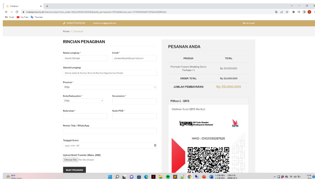
Gambar IV.10 Tampilan Pembayaran
