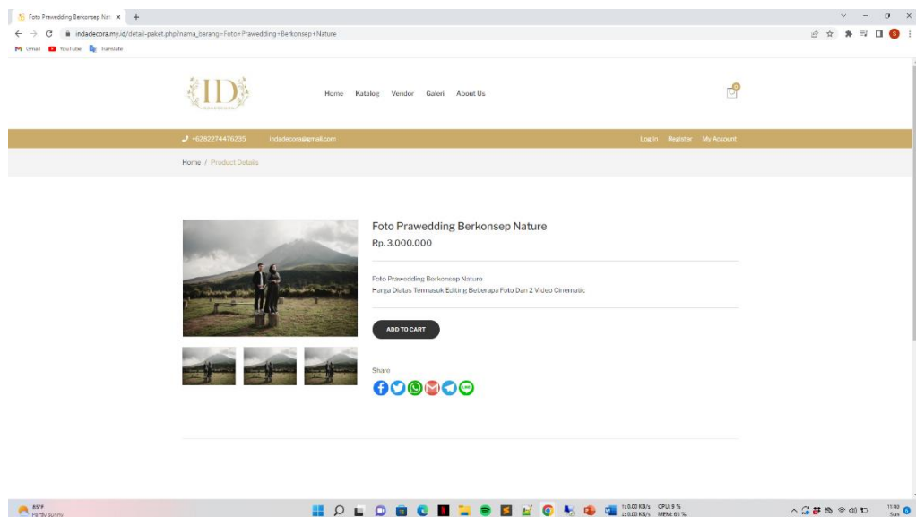
Gambar IV.8 Tampilan Produk
