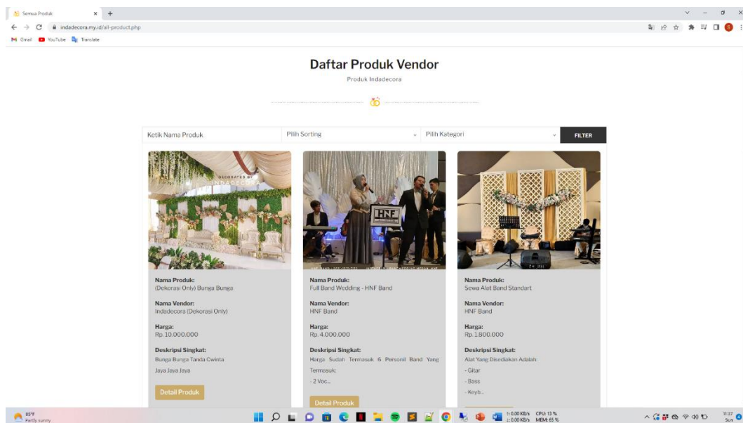
Gambar IV.5 Tampilan Katalog 2
