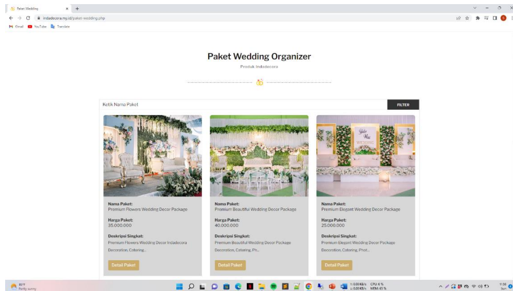
Gambar IV.4 Tampilan Katalog 1
