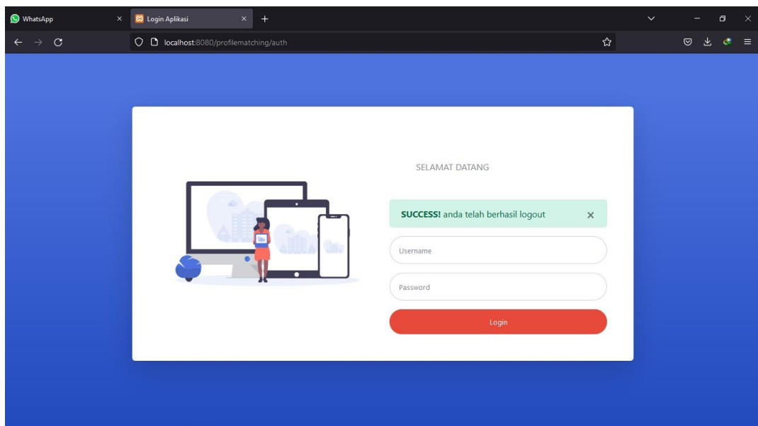
Gambar IV.1 Tampilan Login
