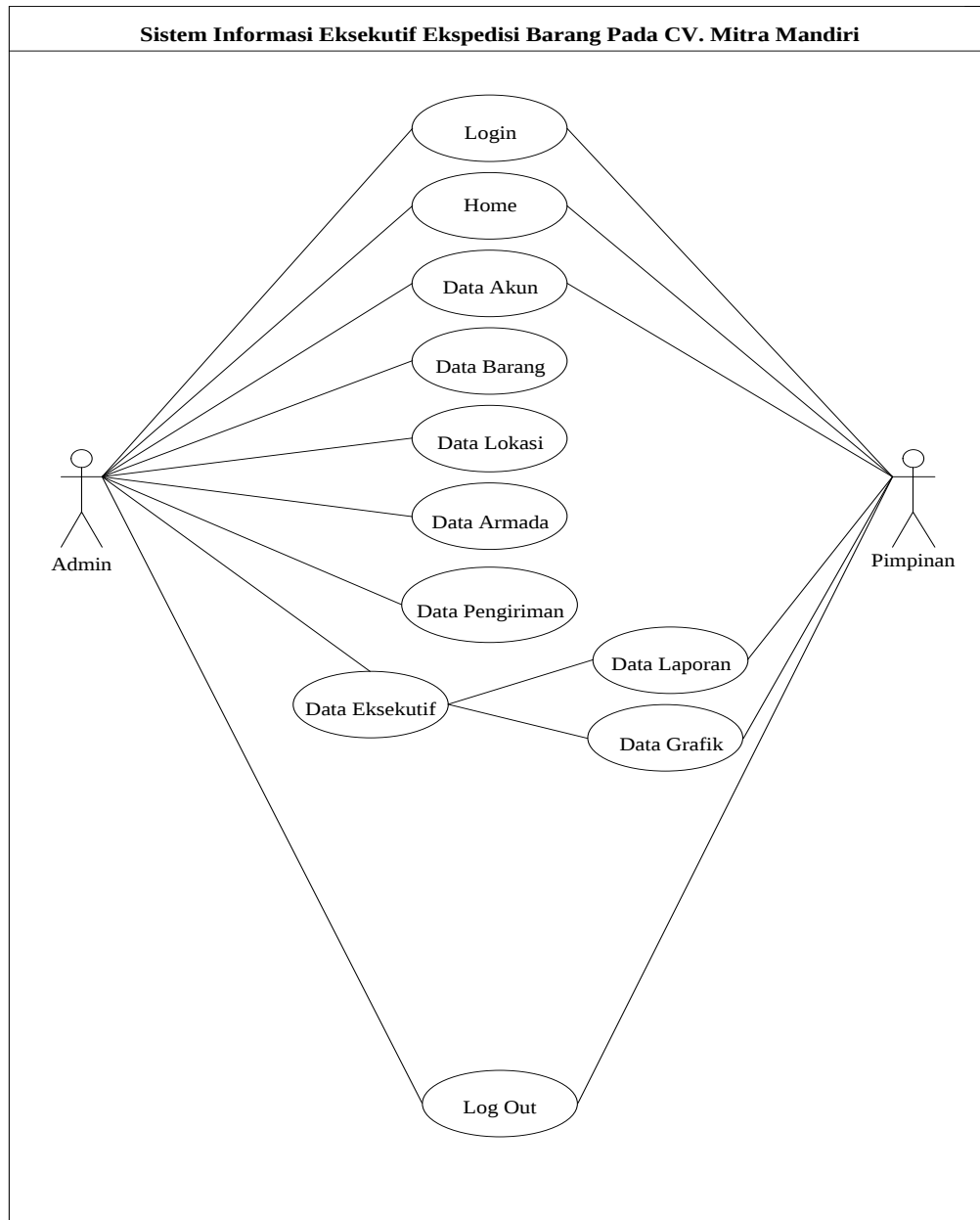
Gambar III.2. Use Case Diagram Sistem Informasi Eksekutif Ekspedisi Barang Pada CV. Mitra Mandiri
