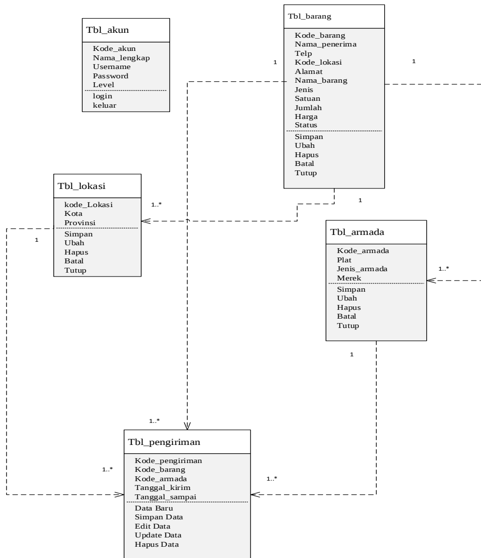
Gambar III.3. Class Diagram Sistem Informasi Eksekutif Ekspedisi Barang Pada CV. Mitra Mandiri
