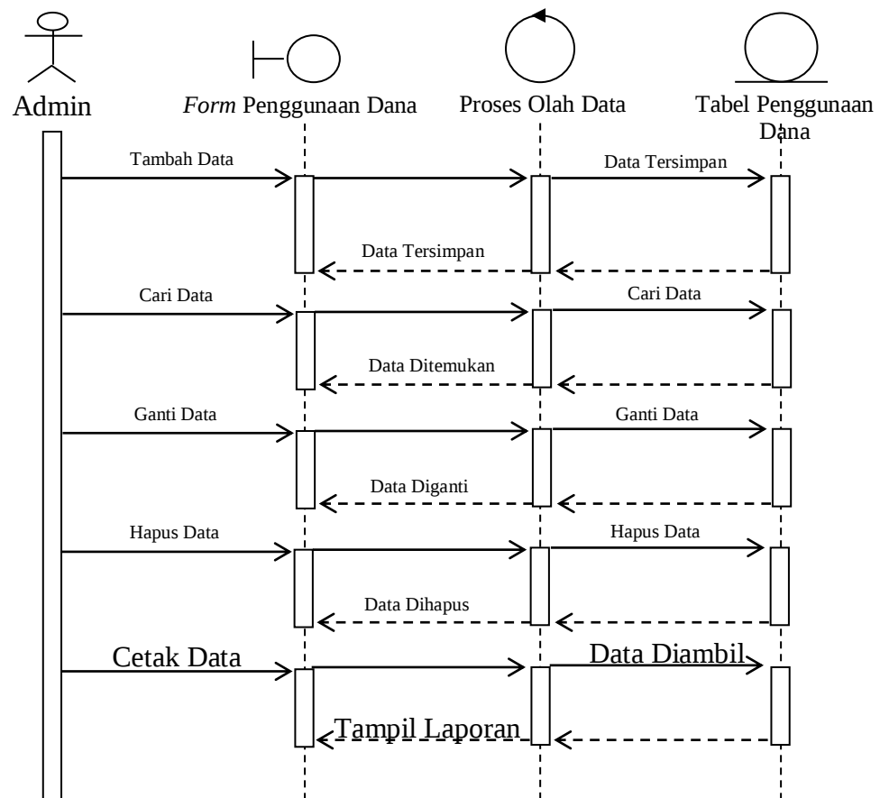
Gambar III.24. Sequence Diagram Penggunaan Dana Bagian Admin
