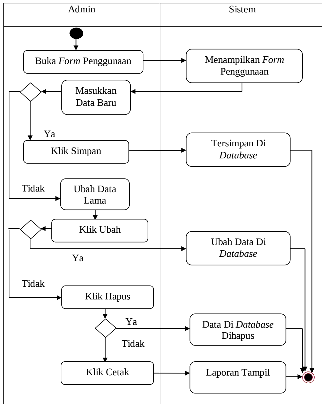
Gambar III.15. Activity Diagram Penggunaan Bagian Admin
