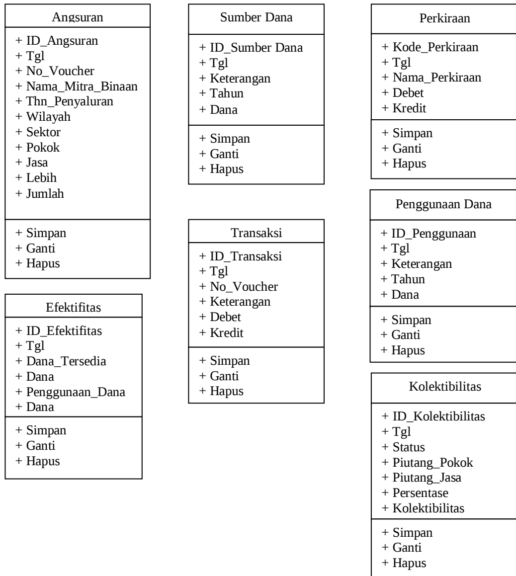
Gambar III.8. Class Diagram Perancangan Aplikasi Monitoring Pembayaran Angsuran Mitra Binaan Pada PT Jasa Marga (Persero) Tbk. Cabang Belmera Berbasis Web
