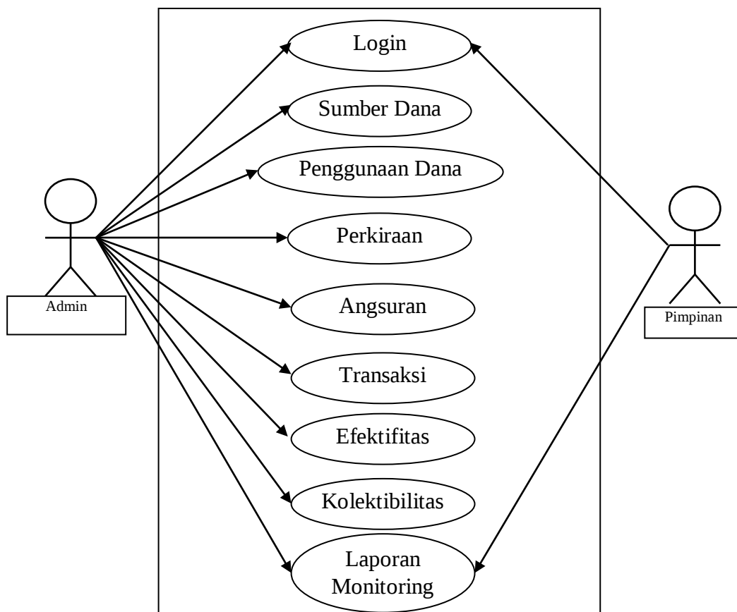
Gambar III.7. Use Case Perancangan Aplikasi Monitoring Pembayaran Angsuran Mitra Binaan Pada PT Jasa Marga (Persero) Tbk. Cabang Belmera Berbasis Web
