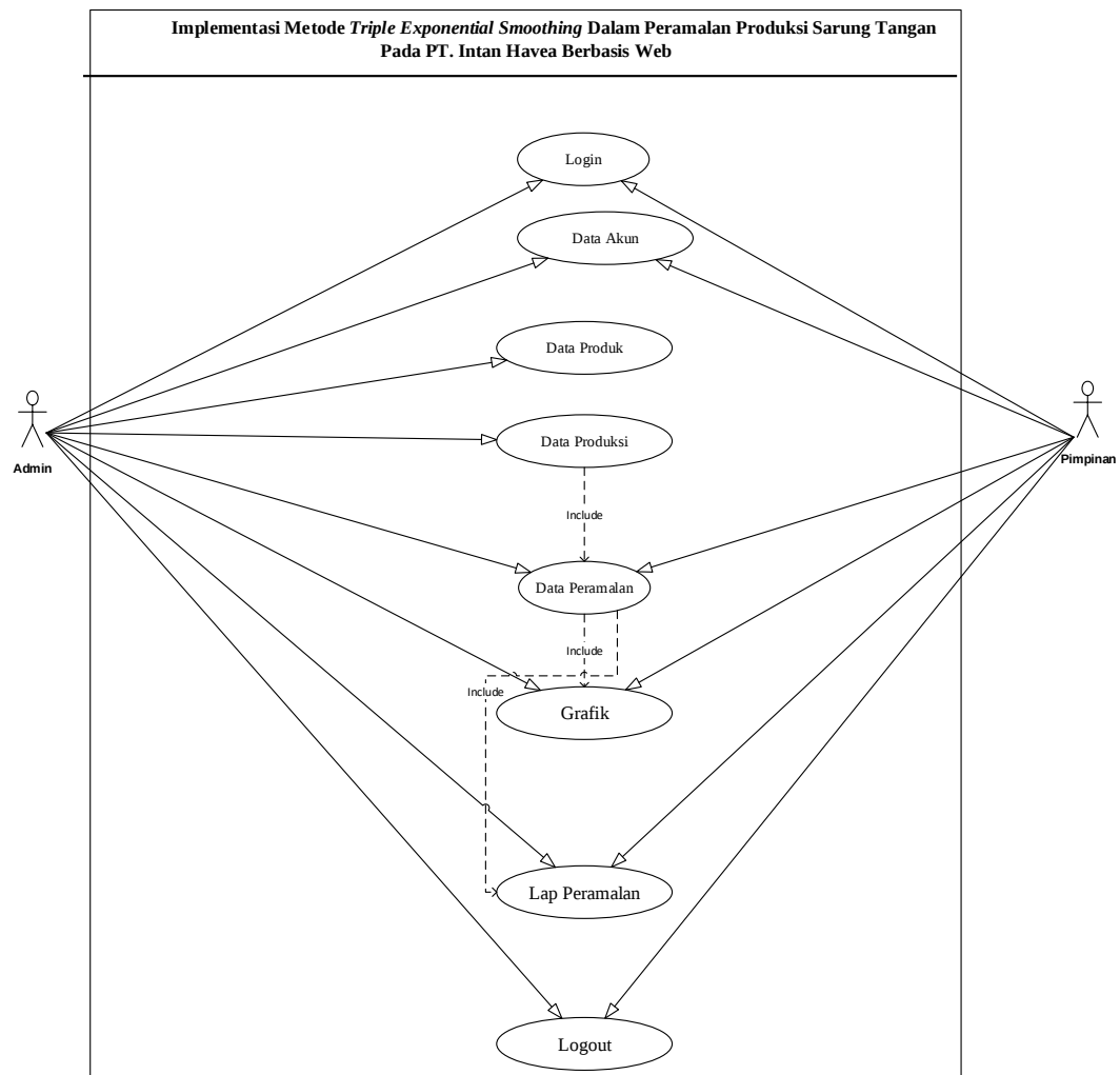
Gambar III.1. Use Case Diagram Implementasi Metode Triple Exponential Smoothing Dalam Peramalan Produksi Sarung Tangan Pada PT. Intan Havea Berbasis Web
