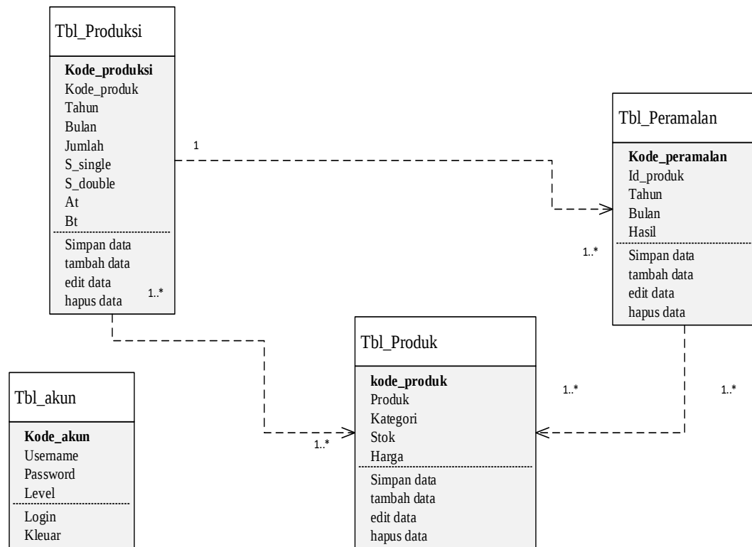
Gambar III.2. Class Diagram Implementasi Metode Triple Exponential Smoothing Dalam Peramalan Produksi Sarung Tangan Pada PT. Intan Havea Berbasis Web
