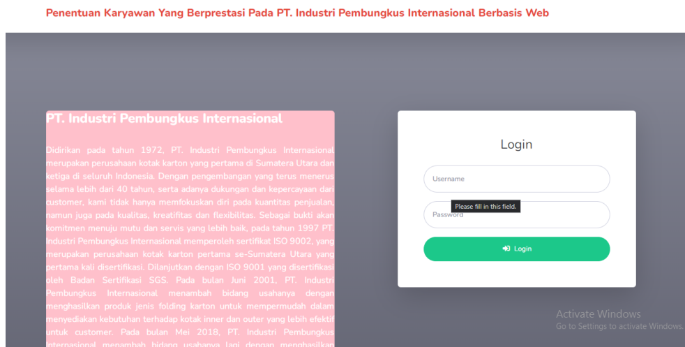
Gambar IV.1 Tampilan Login
