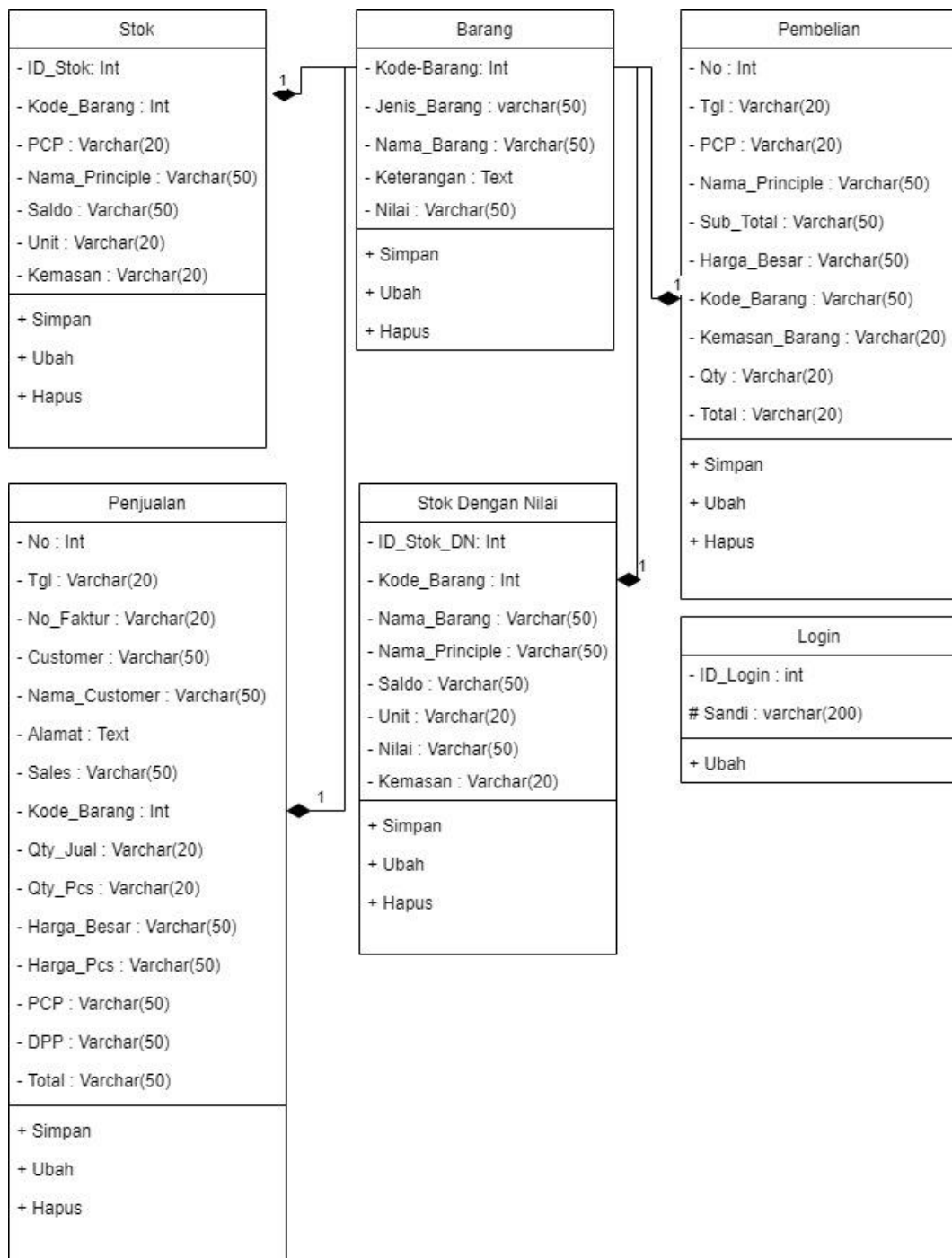
Gambar III.6. Class Diagram Perancangan Sistem Pengolahan Data Pada Distributor PT Sumber Rezeki Bersama Berbasis Web
