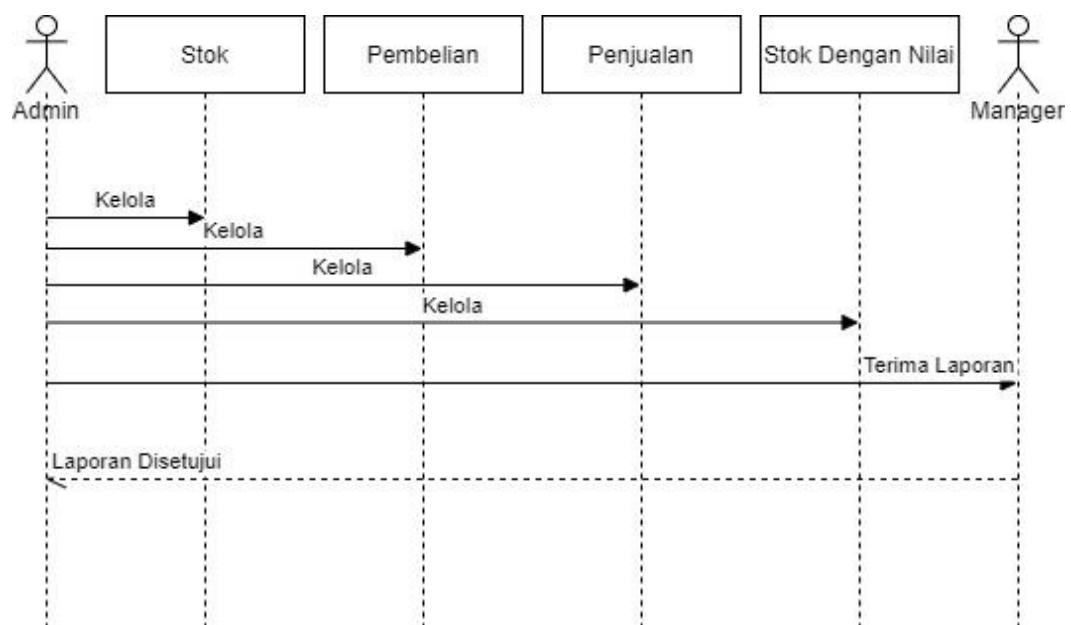
Gambar III.14. Sequence Diagram Sistem Yang Berjalan
