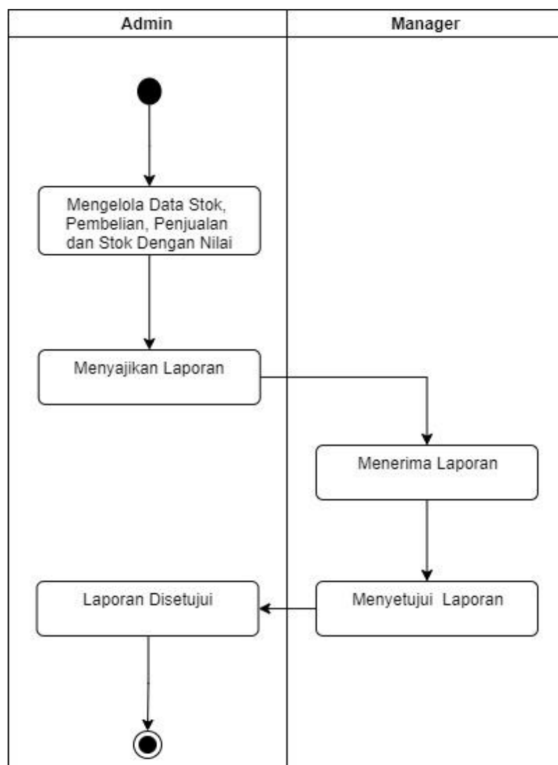
Gambar III.7. Activity Diagram Sistem Yang Berjalan
