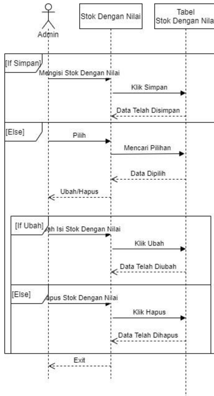
Gambar III.19. Sequence Diagram Stok Dengan Nilai Bagian Admin
