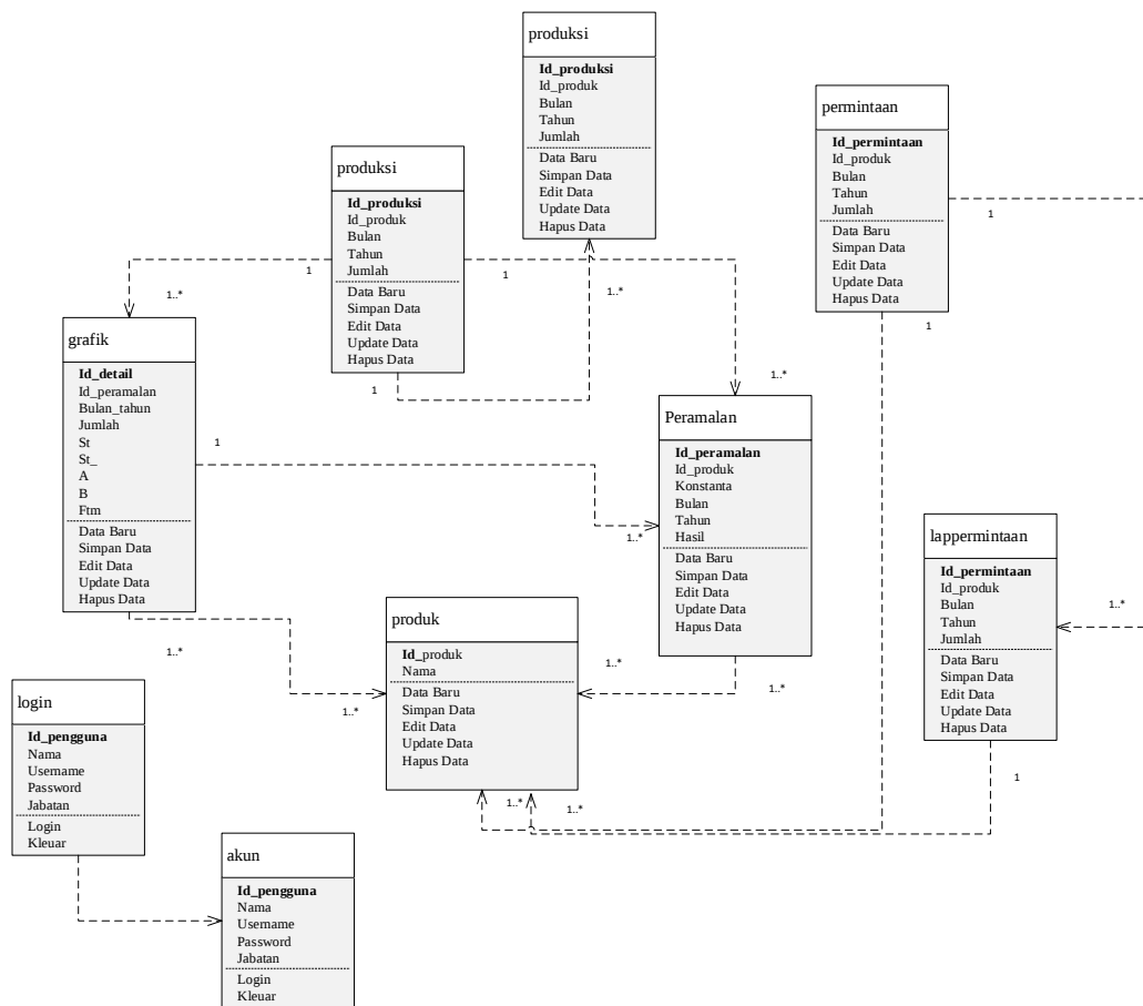
Gambar III.2. Class Diagram Penerapan Metode Trend Projection Dalam Sistem Peramalan Produksi Material Pada PT. Ari Putra Brass Medan berbasis we
