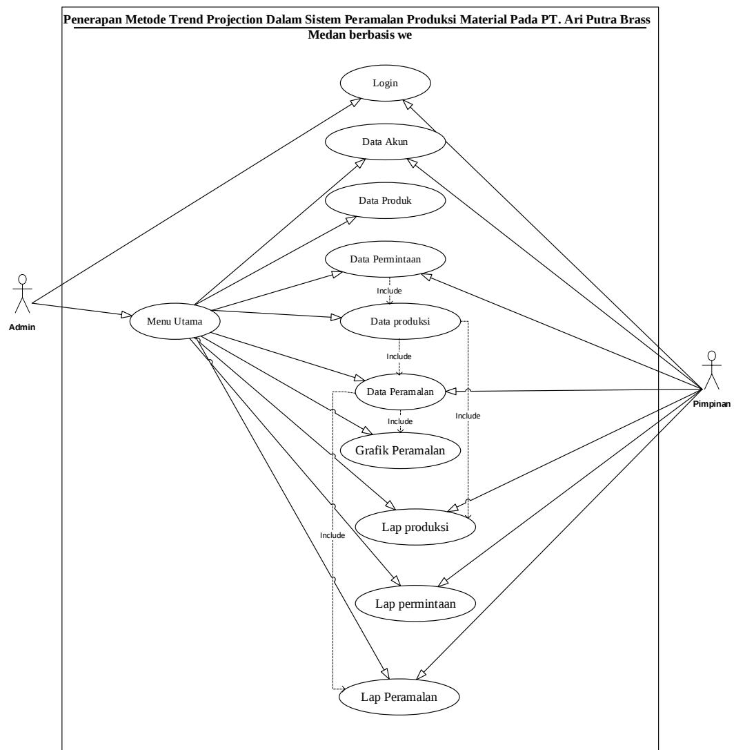
Gambar III.1. Use Case Diagram Penerapan Metode Trend Projection Dalam Sistem Peramalan Produksi Material Pada PT. Ari Putra Brass Medan berbasis we
