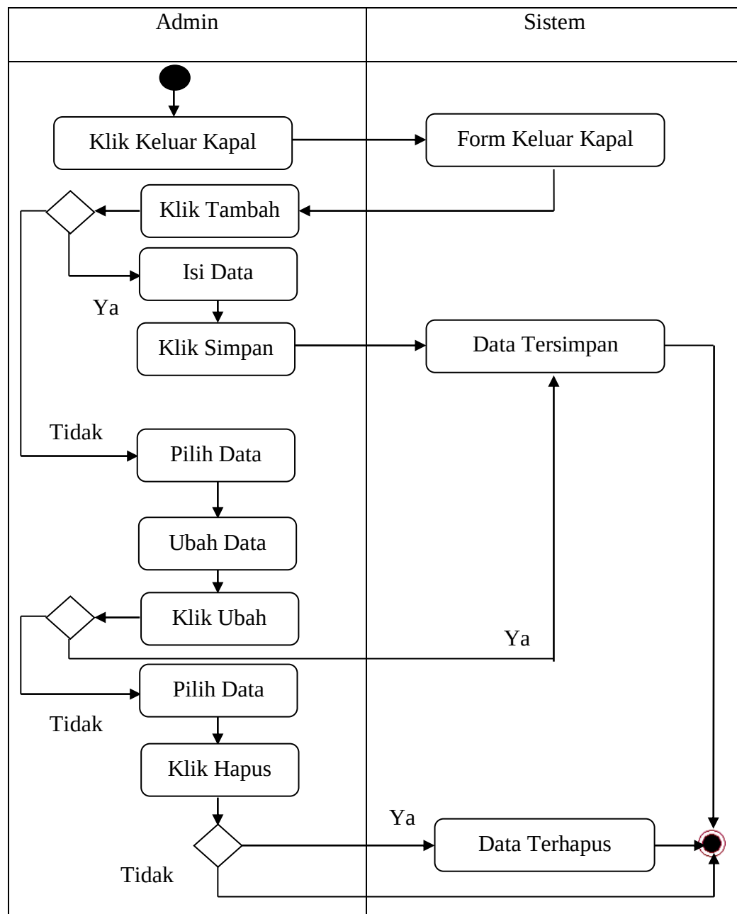
Gambar III.12. Activity Diagram Form Keluar Kapal
