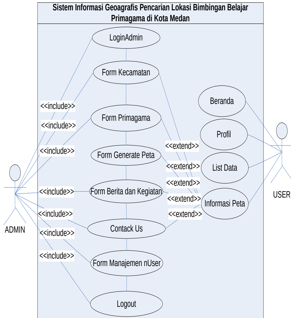
Gambar. III.2 User Case Sistem Informasi Geoagras Pencarian Lokasi Bimbingan Belajar Primagama di Kota Medan
