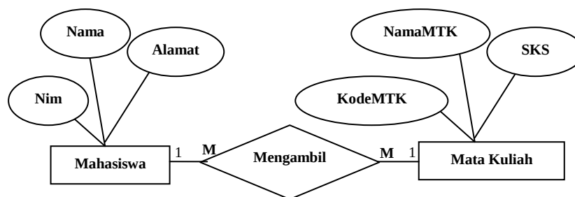
Gambar II.4. Diagram ER
