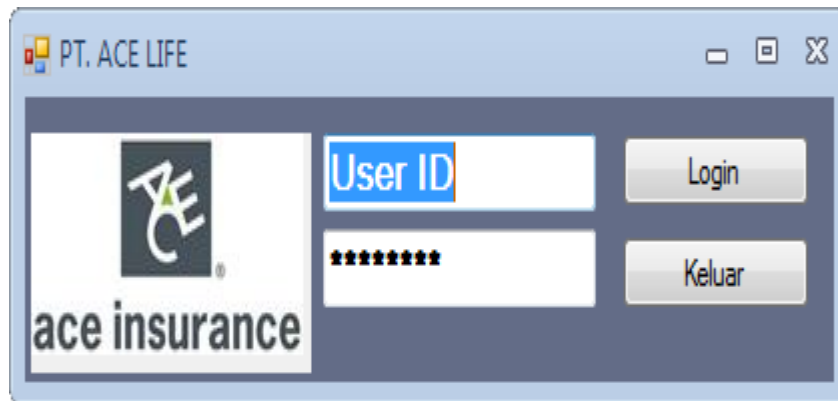
Gambar IV.1. Halaman Login
