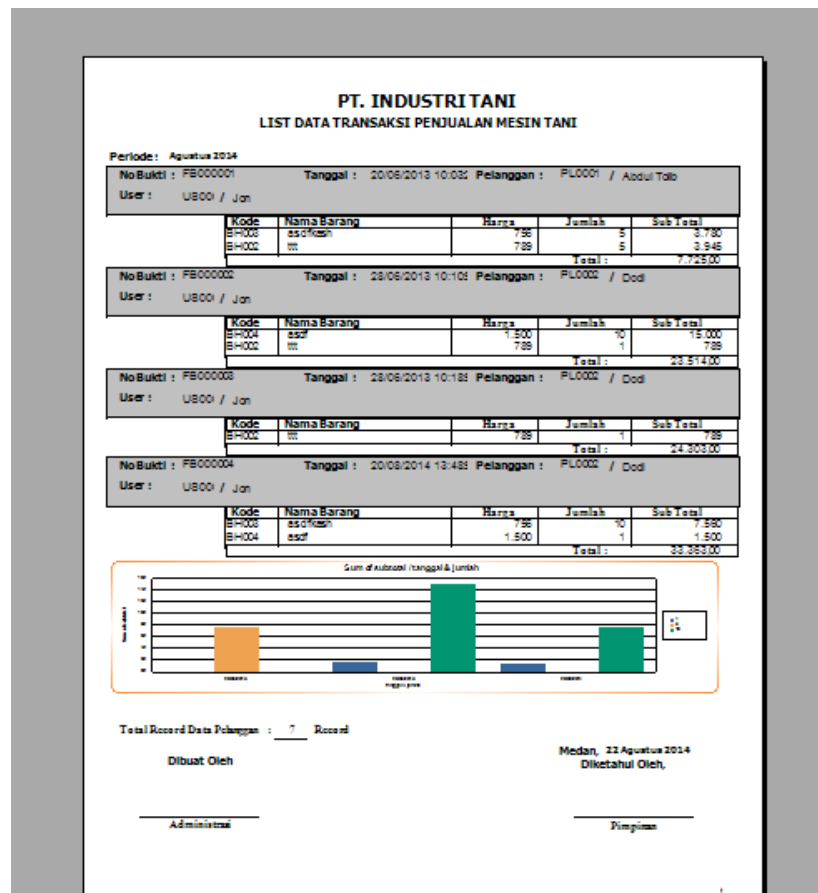
Gambar IV.16. Laporan Penjualan
