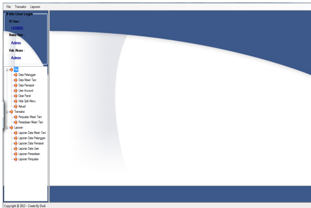
Gambar IV.2.Halaman Menu Utama
