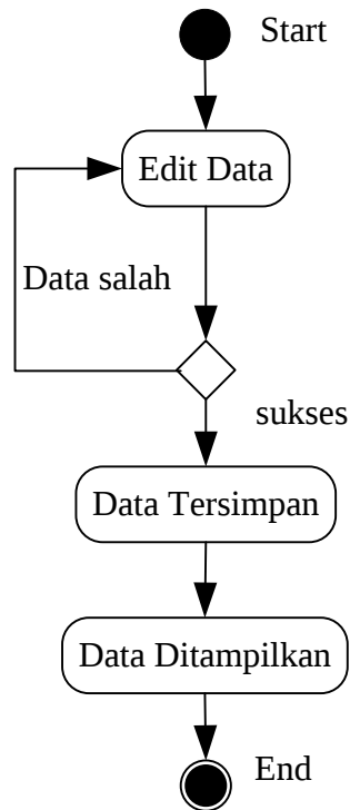
Gambar III.34. Activity Diagram Edit Data Sistem Informasi Geografis Pemetaan Letak Ruangan pada Badan Pusat Statistik Provinsi Sumatera Utara
