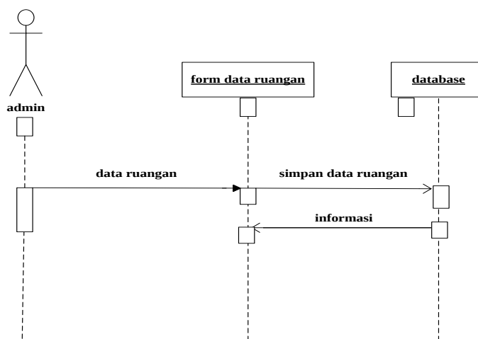
Gambar III.6. Sequence Diagram pada Form Data Ruangan
