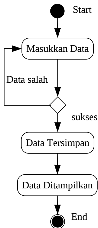
Gambar III.33. Activity Diagram Input Data Sistem Informasi Geografis Pemetaan Letak Ruangan pada Badan Pusat Statistik Provinsi Sumatera Utara
