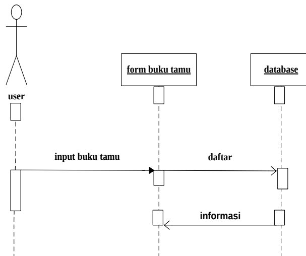
Gambar III.9. Sequence Diagram pada Form Data Buku Tamu
