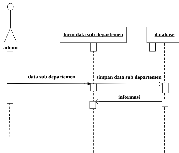
Gambar III.5. Sequence Diagram pada Form Data Sub Departemen
