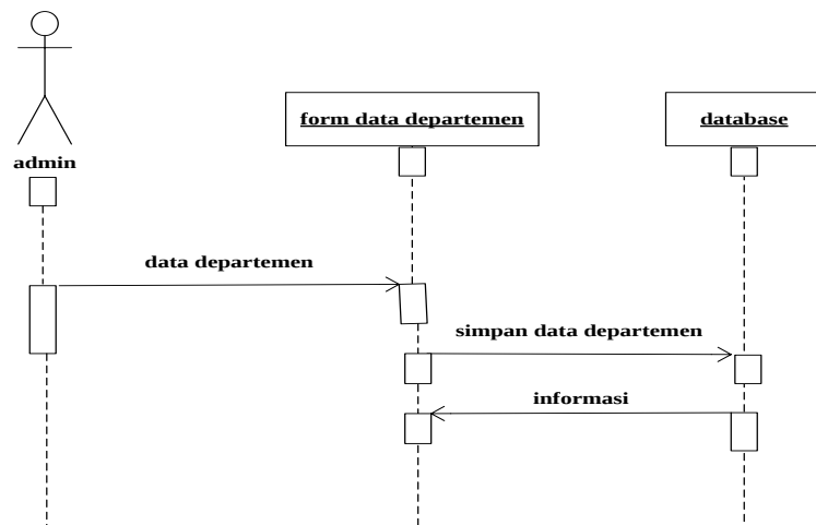
Gambar III.4. Sequence Diagram pada Form Data Departemen
