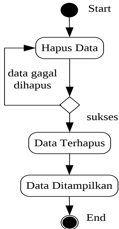
Gambar III.35. Activity Diagram Hapus Data Sistem Informasi Geografis Pemetaan Letak Ruangan pada Badan Pusat Statistik Provinsi Sumatera Utara
