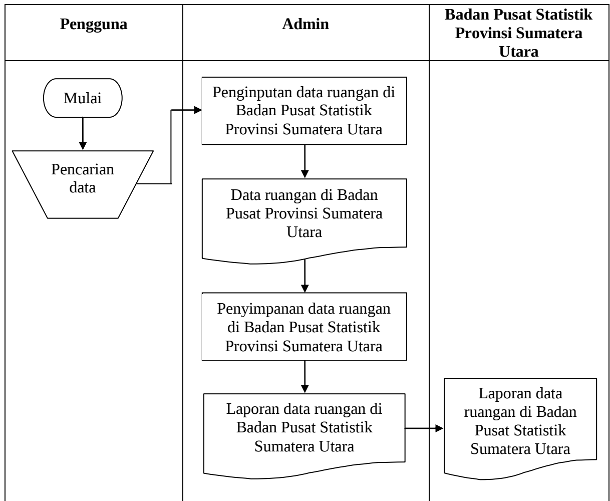
Gambar III.1. FOD Penyimpanan Data
