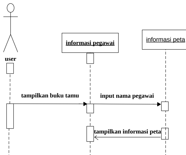
Gambar III.12. Sequence Diagram pada Form Pencarian Informasi
