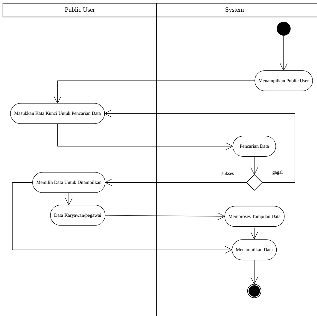
Gambar III.37. Activity Diagram Pencarian Data Sistem Informasi Geografis Pemetaan Letak Ruangan pada Badan Pusat Statistik Provinsi Sumatera Utara
