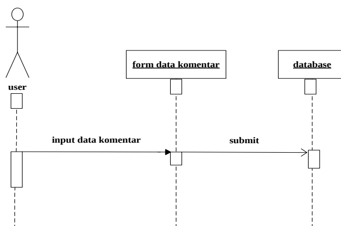
Gambar III.8. Sequence Diagram pada Form Data Komentar
