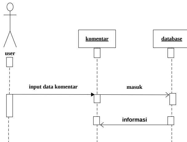
Gambar III.10. Sequence Diagram pada Form Data User Khusus
