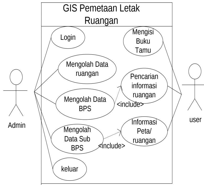
Gambar III.2. Usecase Diagram Sistem Informasi Geografis Pemetaan Letak Ruangan pada Badan Pusat Statistik Provinsi Sumatera Utara
