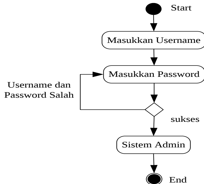
Gambar III.32. Activity Diagram Login Admin Sistem Informasi Geografis Pemetaan Letak Ruangan pada Badan Pusat Statistik Provinsi Sumatera Utara
