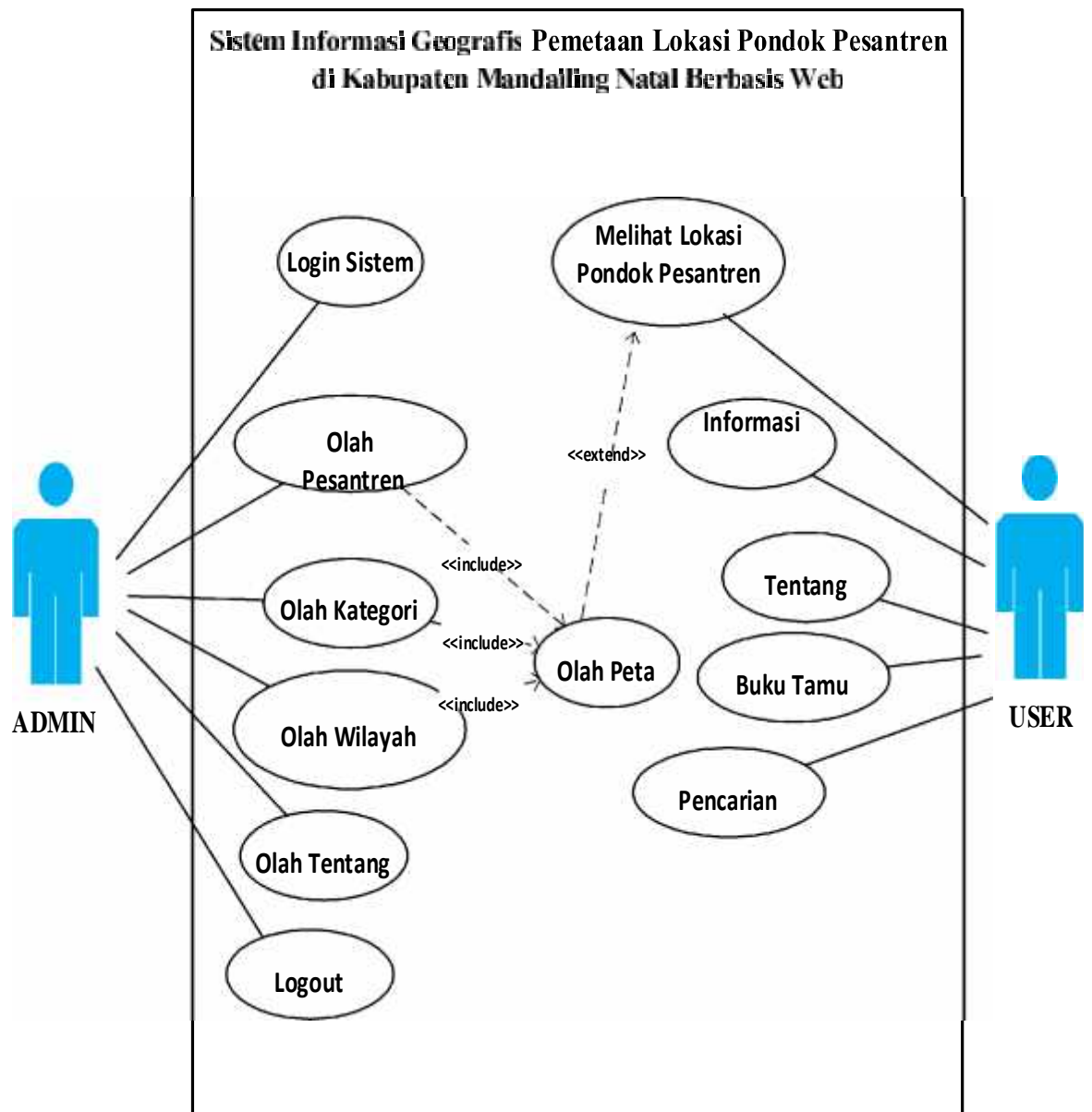
Gambar III.1. Use Case Diagram Sistem Informasi Geografis Lokasi Pondok Pesantren di Kabupaten Mandailing Natal
