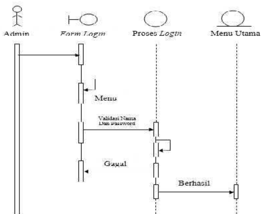
Gambar III.9. Sequence Diagram Pada Halaman Login
