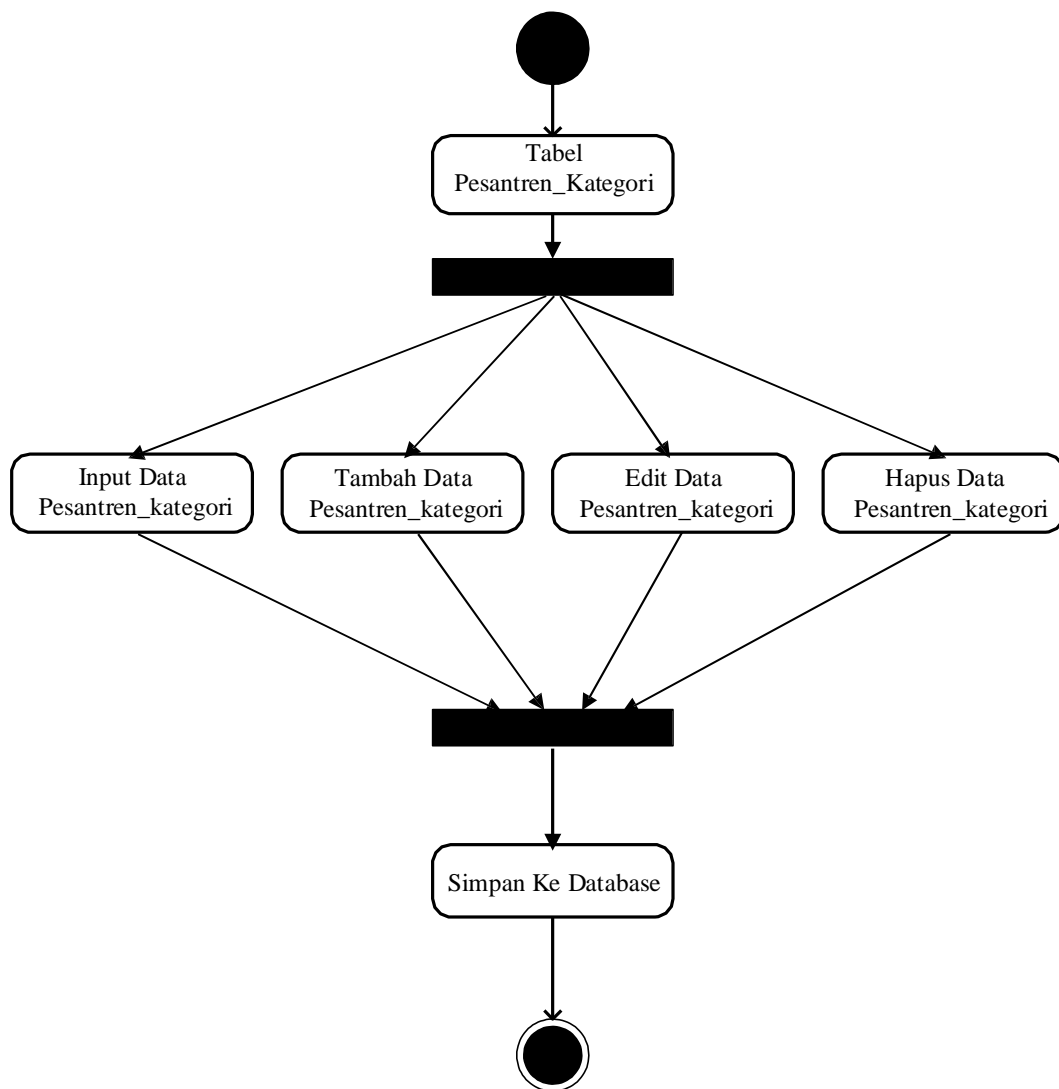
Gambar III.7. Activity Diagram Tabel Pesantren_Kategori Sistem Informasi Geografis Lokasi Pondok Pesantren di Kabupaten Mandailing Natal
